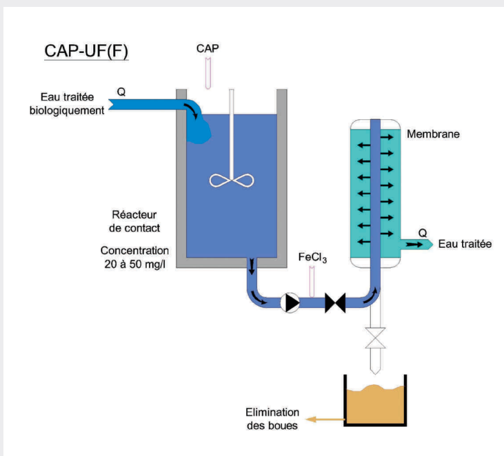
Fig. 4 Schéma simplifié du procédé CAP-UF(F)
