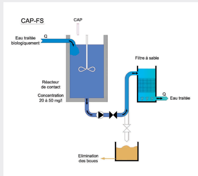
Fig. 3 Schéma simplifié du procédé CAP-FS Vereinfachtes Schema des Prozesses PAK-SF
