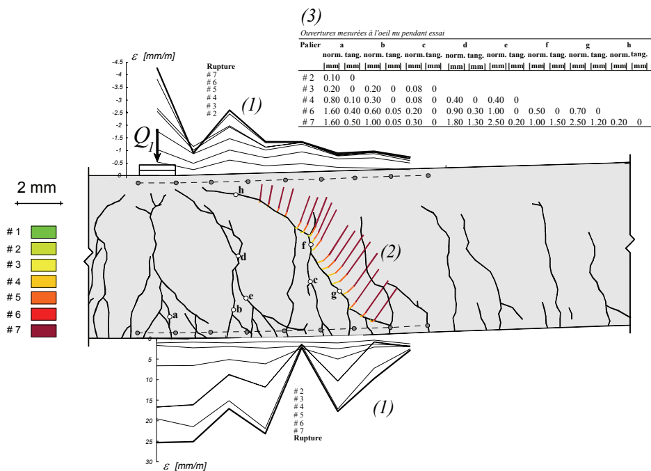
Figure B-4.17: Poutre SR4: (1) Déformations mesurées avec les jauges “oméga” ; (2) Déplacement relatif entre les 2 lèvres des fissures, calculé avec les mesures au déformètre; (3) Ouvertures mesurées à l’œil nu pendant l’essai
