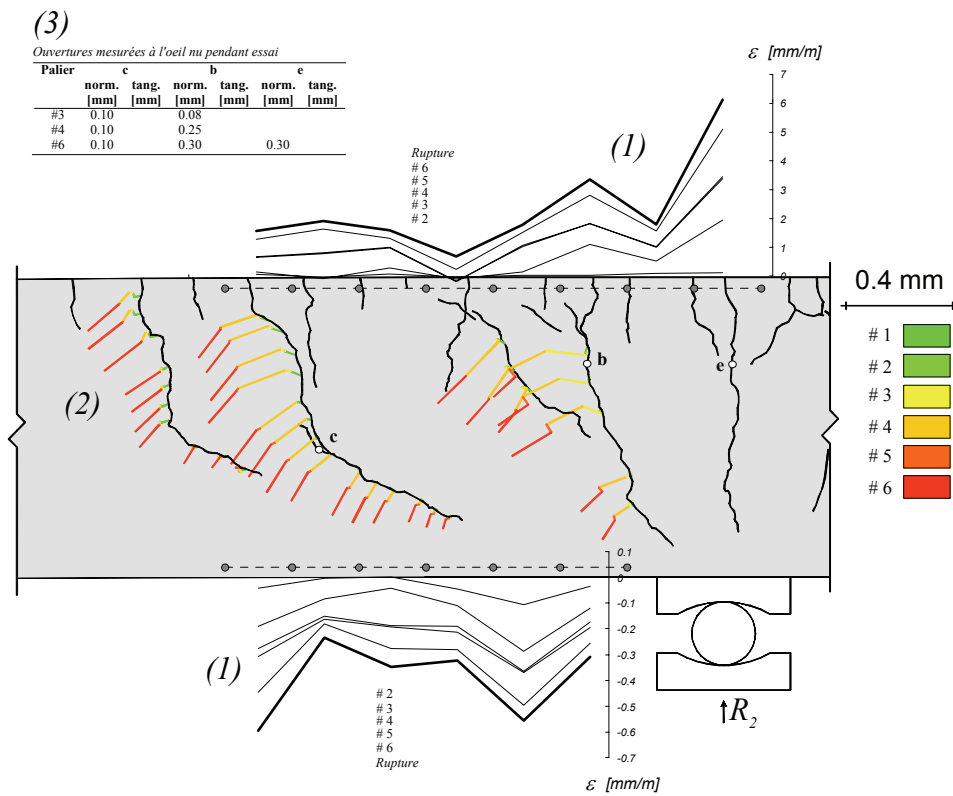
Figure B-4.7: (1) Déformations mesurées avec les jauges "oméga"; (2) Déplacement relatif entre les 2 lèvres des fissures, calculé avec les mesures au déformètre; (3) Ouvertures mesurées à l'œil nu pendant l'essai
