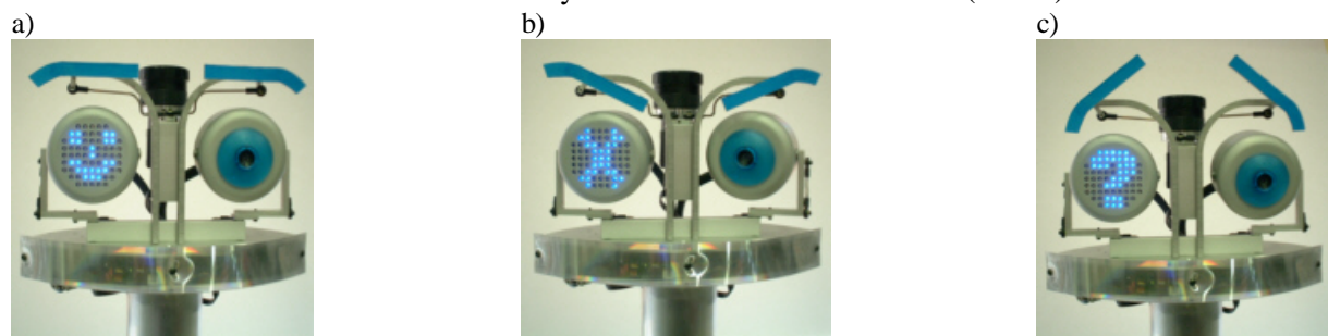
Bild 2 Von RoboX imitierte Gesichtsausdrücke a) neutral freundlich, b) verärgert, c) überrascht.
