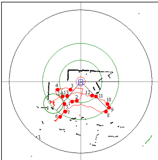
Bild 3 a) Bewegungsdetektion mittels Laser Scanner Daten. Der Roboter ist in der Bildmitte zu sehen. Die konzentrischen Kreise zeigen die verschiedenen Sektoren (nah, weit, zu weit). Die beiden diagonalen Linien grenzen den linken, den vorderen und den rechten Sektor voneinander ab. Der äußerste Kreis entspricht dem Sensorhorizont (8 m), Punkte, die ausserhalb liegen, wurden als nicht zuverlässige Messungen klassifiziert. Die durchgezogene Linie ist die Bewegungstrajektorie des Besuchers. Der kleine Kreis links unten im Bild gibt die Akzeptanz Region für die nächsten Messungen an. b) Von RoboX generierte Kommentare zur Bewegung des Besuchers.
