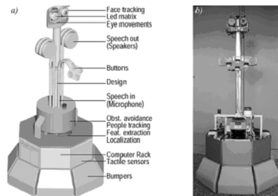
Bild 1: a) Elemente des interaktiven Roboters RoboX, b) der erste Prototyp.
