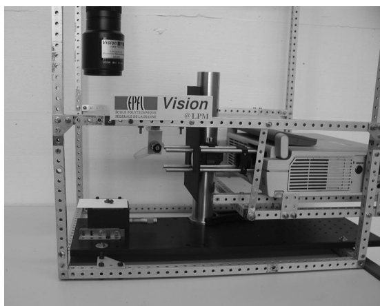
Fig. 8: Notre appareil de laboratoire. On distingue le beamer à droite, l'objectif télécentrique monté sur des rails optiques, le miroir oblique, le plan de pose (en clair) au dessus duquel est placée la caméra.
