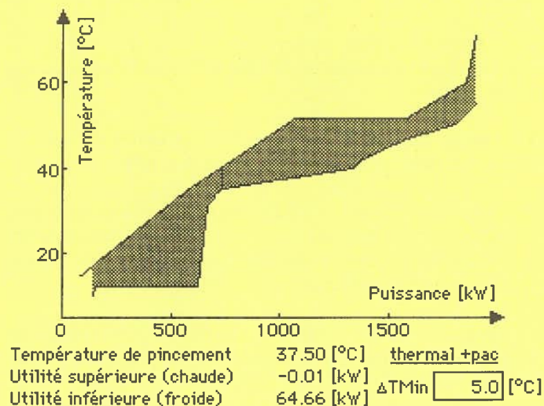
Figure 10b: Composites de l'établissement thermal avec pompe à chaleur seule.
