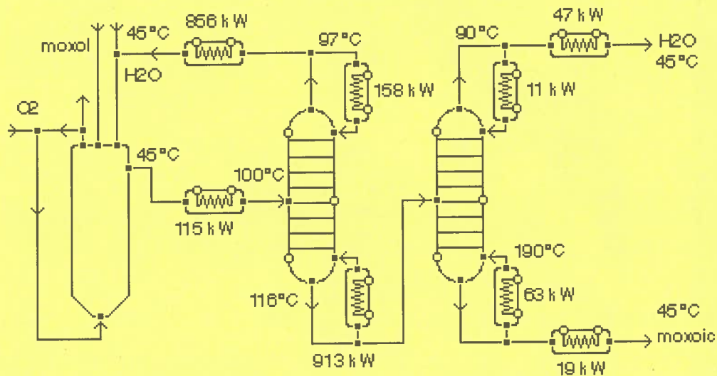
Figure 7: Schéma simplifié du procédé de fabrication de l'acide méthoxyacétique.
