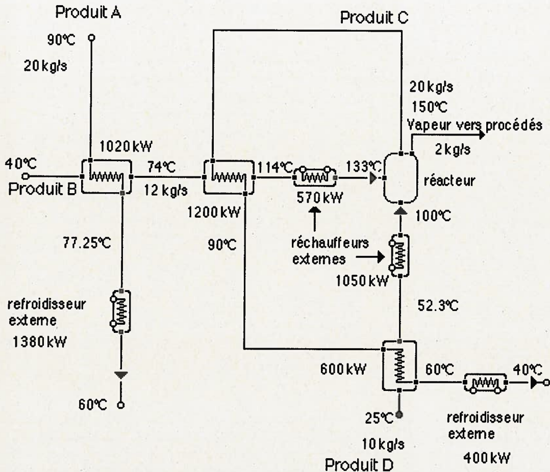
Figure 4a: Exemple de site de production d'un composé chimique.
