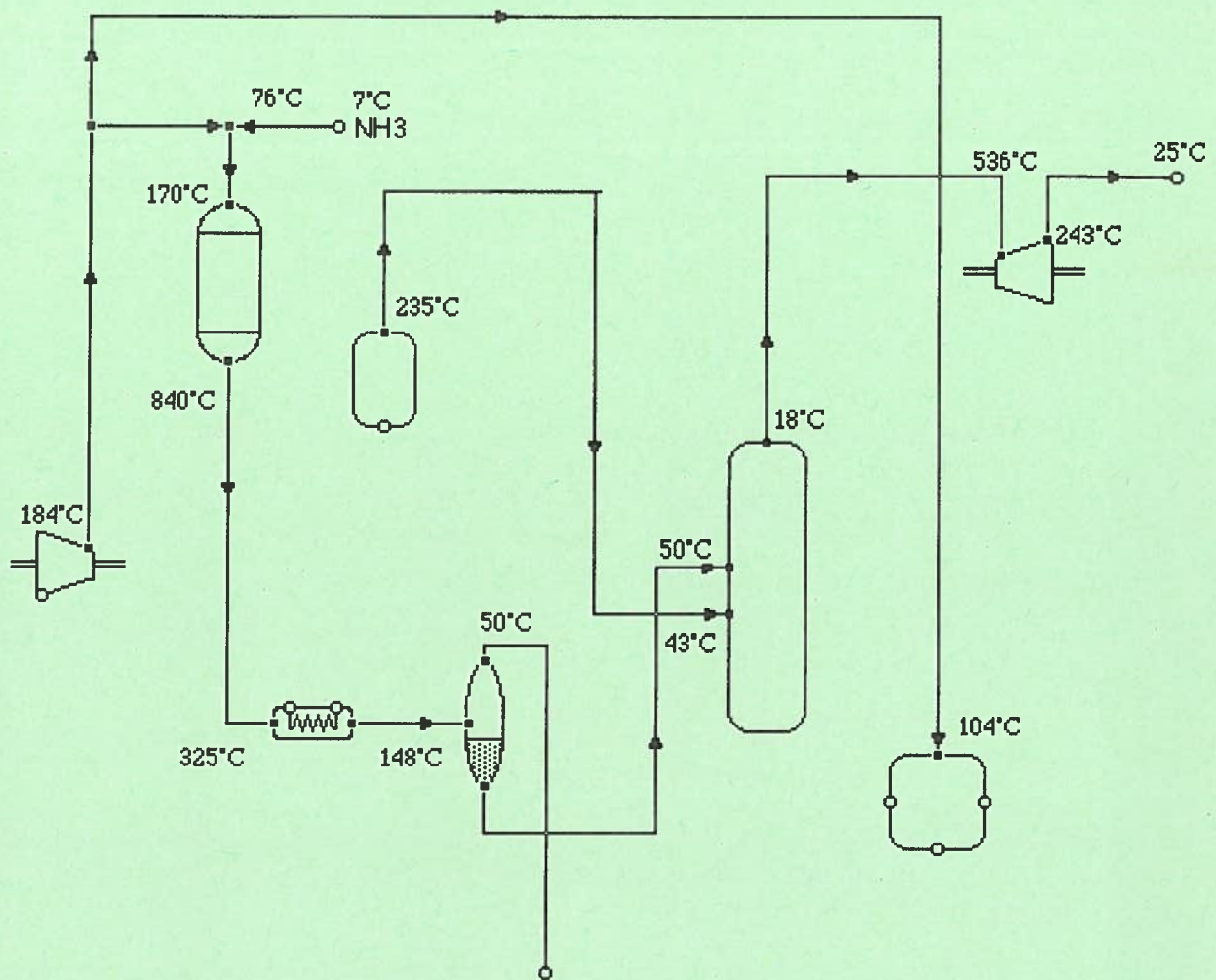
Abb 2b: Wichtigste Aufgaben einer Salpetersäureanlage (vereinfachtes Schema).
