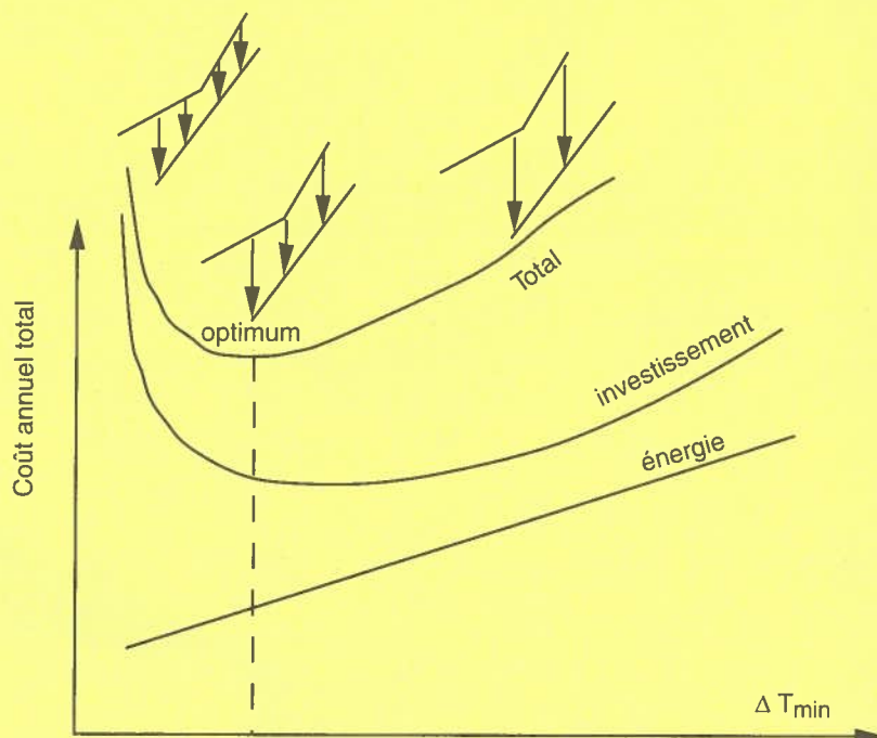
Figure 5: Evolution des différents coûts en fonction du \Delta T_{min} .
