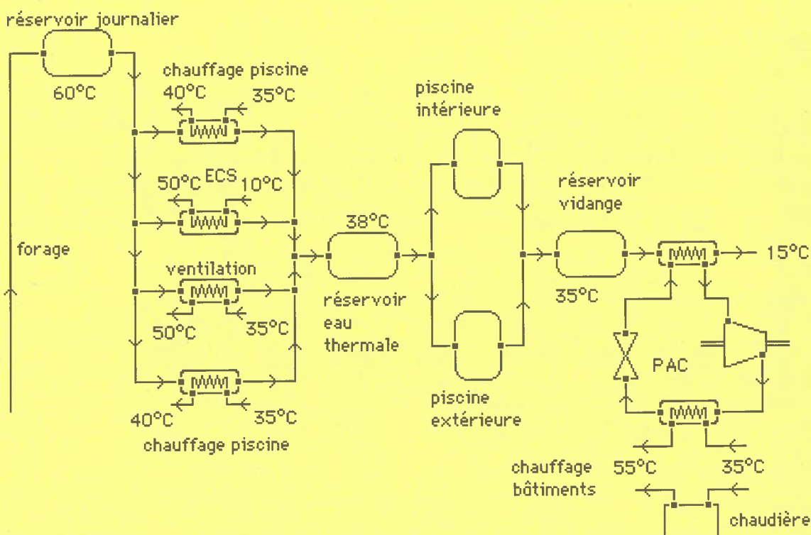
Figure 9 : Schéma simplifié des réseaux de distribution de l'établissement thermal.
