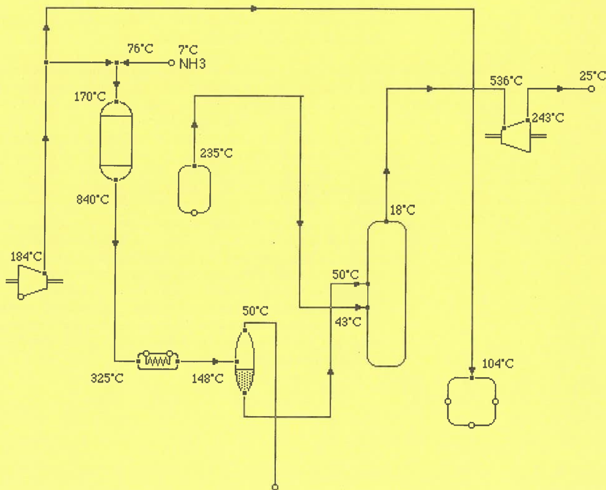
Figure 2b: Diagramme simplifié (cahier des charges) d'une installation de production d'acide nitrique.
