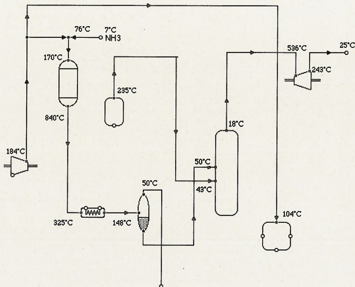
Figure 3b: Diagramme simplifié (cahier des charges) d'une installation de production d'acide nitrique.
