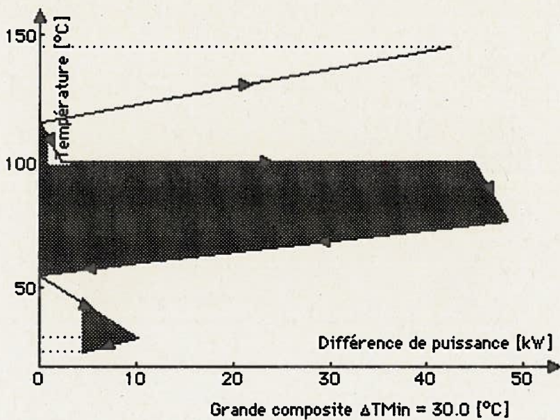
Figure 31: Introduction d'un apport de vapeur à 115°C (100°C dans le diagramme de la grande composite) dans le cas de la figure 30c. Apparition d'un pincement externe.
