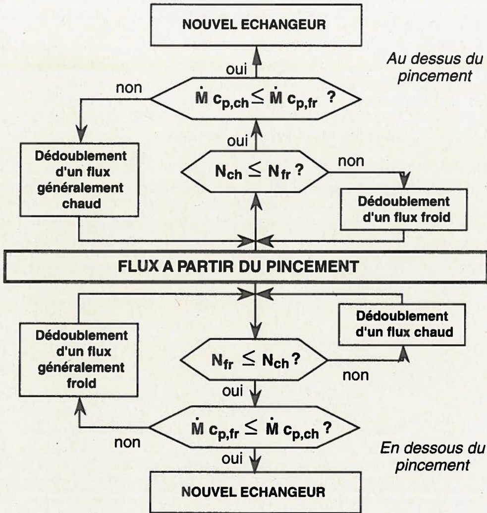
Figure 24 : Organigramme de conception du réseau à consommation d'énergie minimum.
