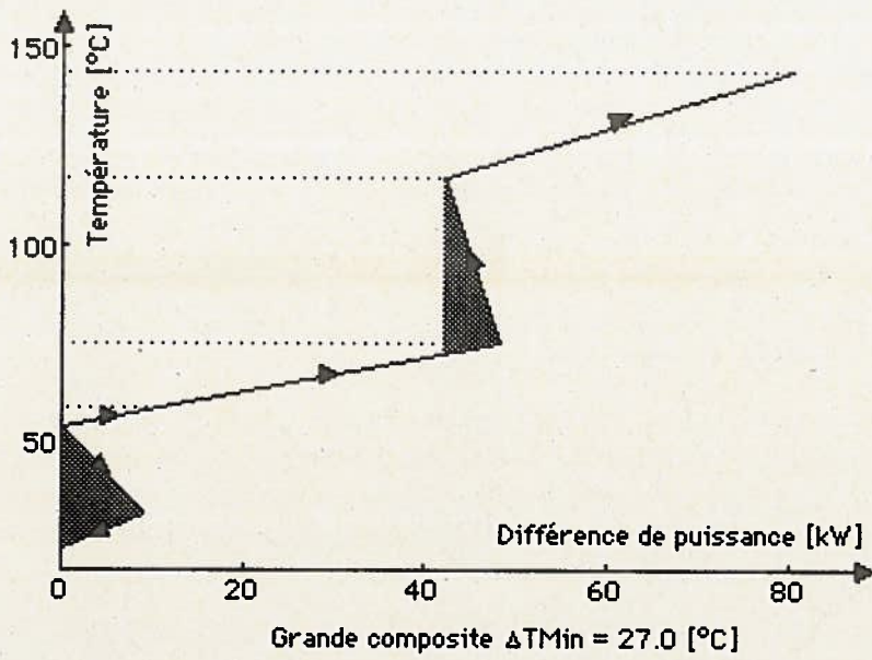
Figure 30b: Grande composite relative au cas limite de la table 2 avec \Delta T_{\min} = 27^{\circ}\text{C} .
