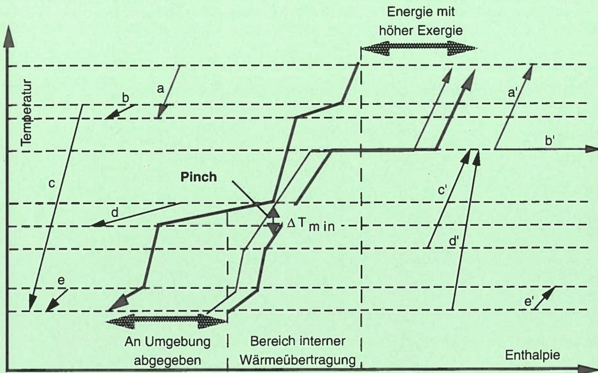
Abb. 3: Stromvektoren und Composite Curves in einem Temperatur - Enthalpie Diagramm.
