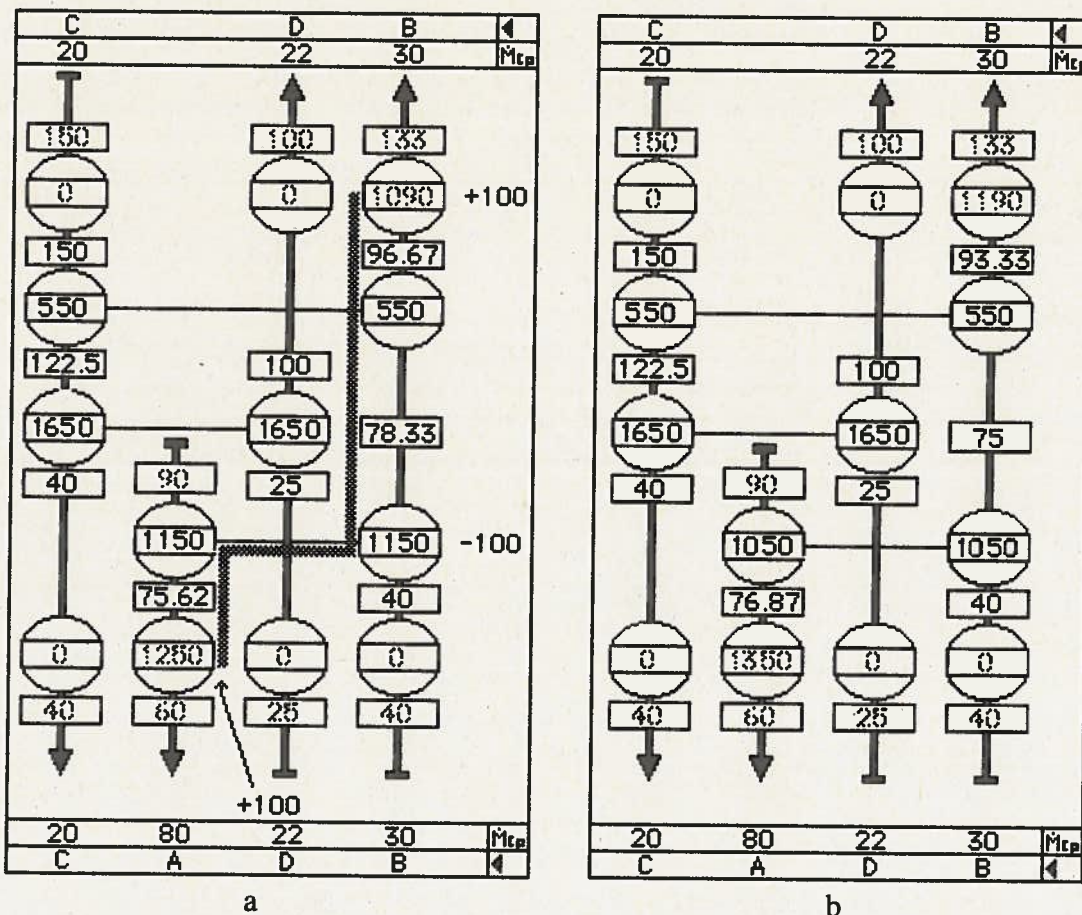
Figure 20: Réseau après suppression de deux boucles (a) et après correction finale (b).
