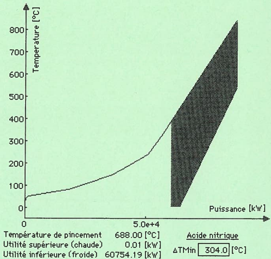
Abb. 4a: Composite Curves der Salpetersäureproduktion.
