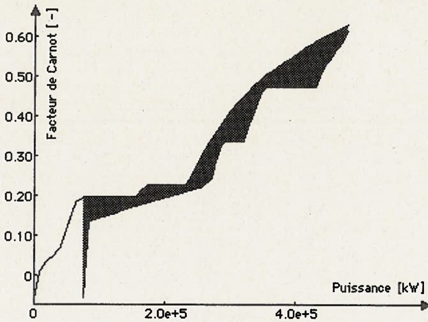
Figure 36: Courbes composites d'une centrale à cycle combinée.
