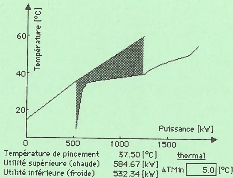
Abb. 10a: Den Rahmenbedingungen des Thermalbades entsprechende Composite Curves.
