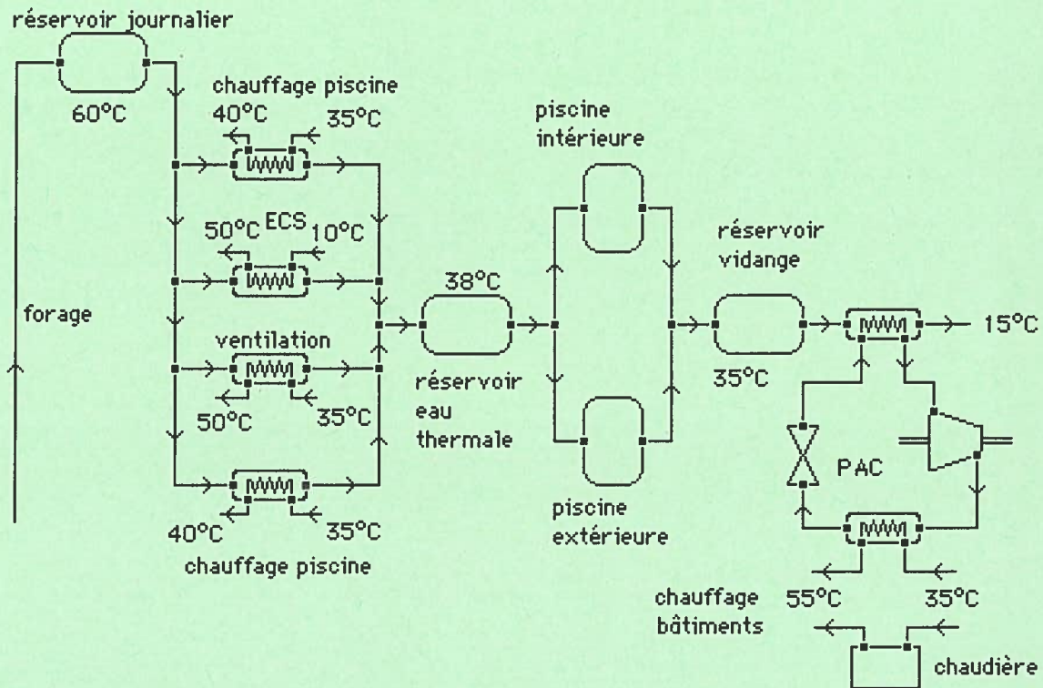
Abb. 9: Vereinfachtes Schema des Heizungssystems des Thermalbades.
