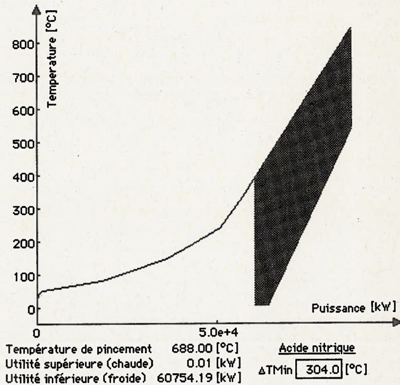
Figure 12a: Composites de l'installation d'acide nitrique seule.
