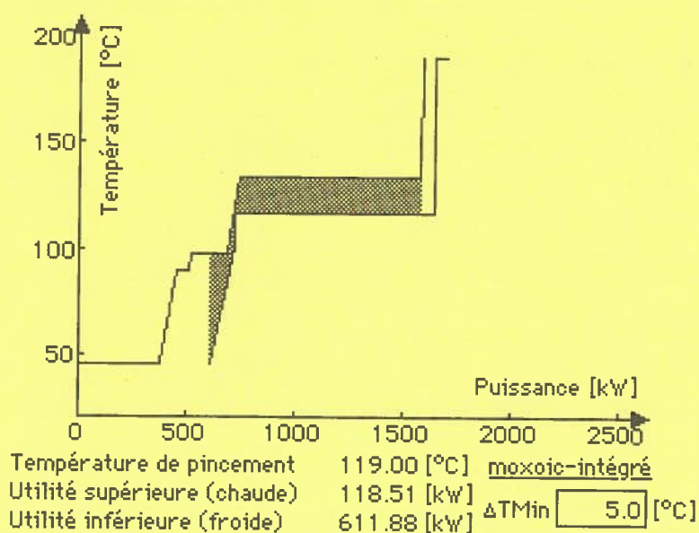
Figure 8b: Composites du procédé de fabrication de l'acide méthoxyacétique avec intégration d'une recompression mécanique de vapeurs.
