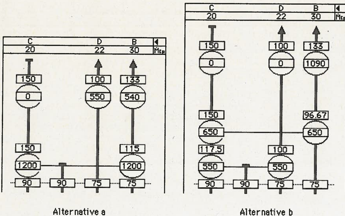
Figure 14: Alternatives de réseaux à consommation d'énergie minimum pour la zone puits.
