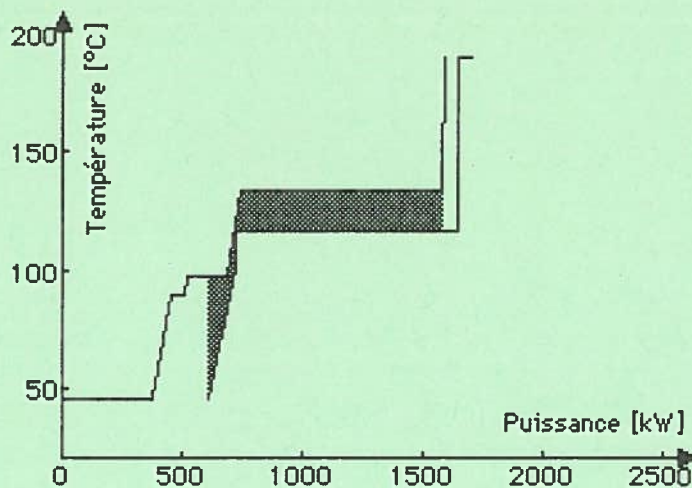
Abb. 8a: Ursprüngliche Composite Curves des Prozesses Methoxyessigsäure.
