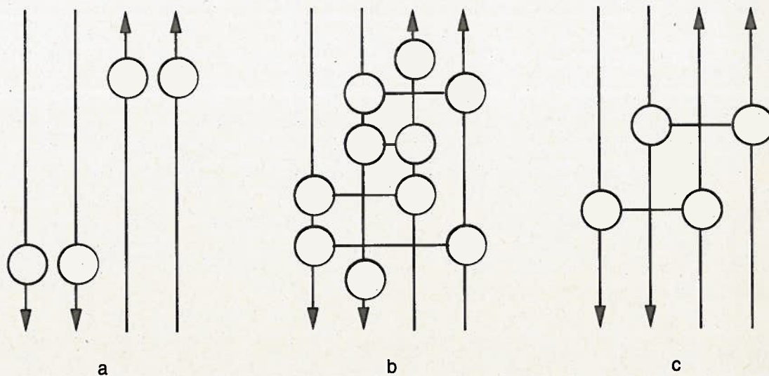
Figure 2: Solutions possibles de réseaux d'échange pour un site simplifié à quatre flux.
