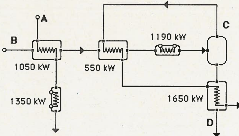
Figure 22: Version améliorée du réseau d'échangeurs du procédé de la figure 4a.
