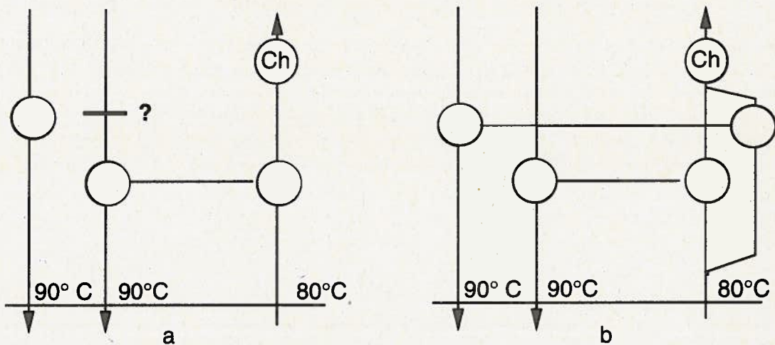
Figure 23 : Dédoublage par déséquilibre du nombre de flux.
