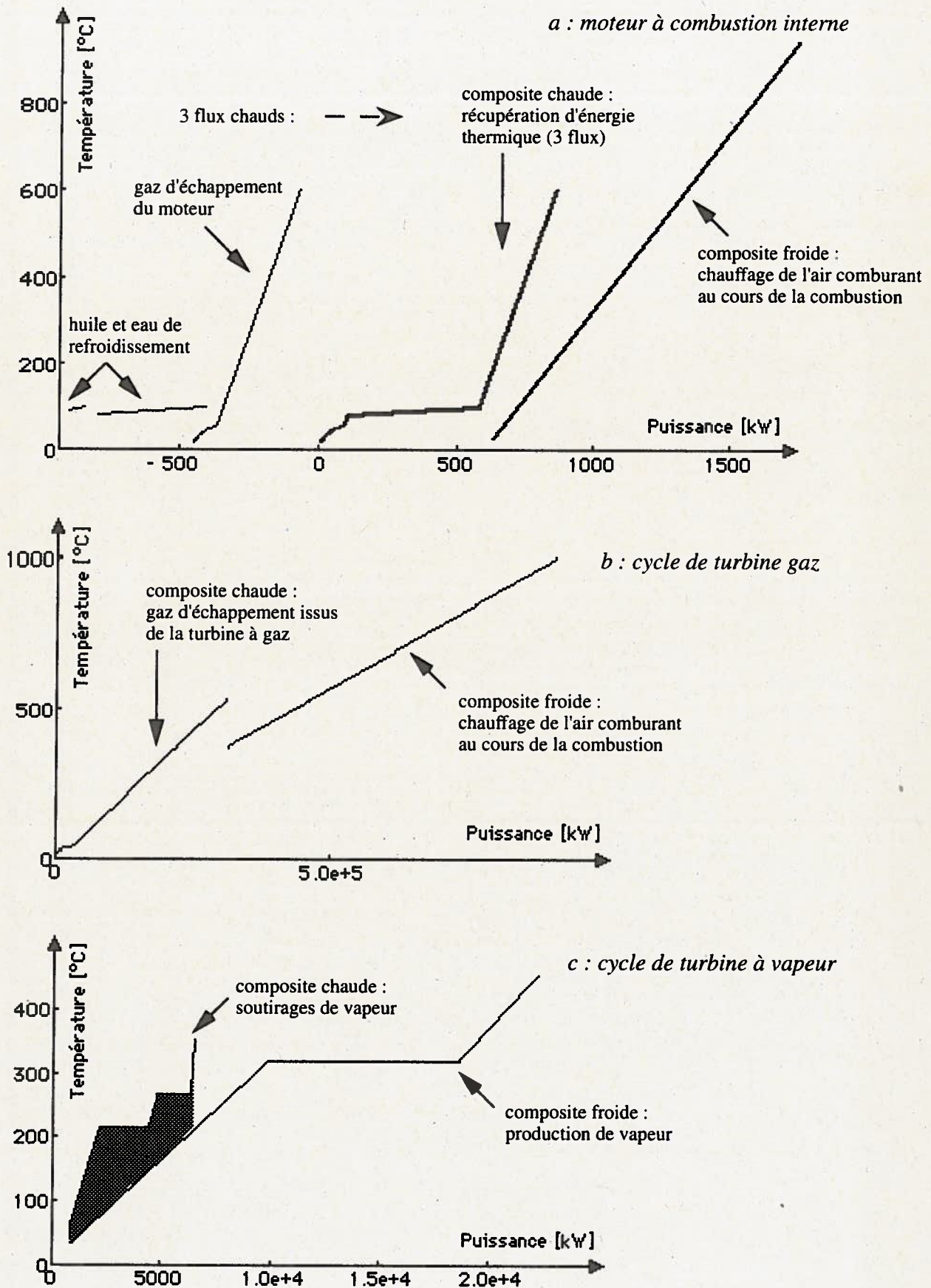
Figure 34 : Courbes composites relatives aux techniques de cogénération (a : moteur à combustion interne, b : cycle de Brayton, c : cycle de Rankine).
