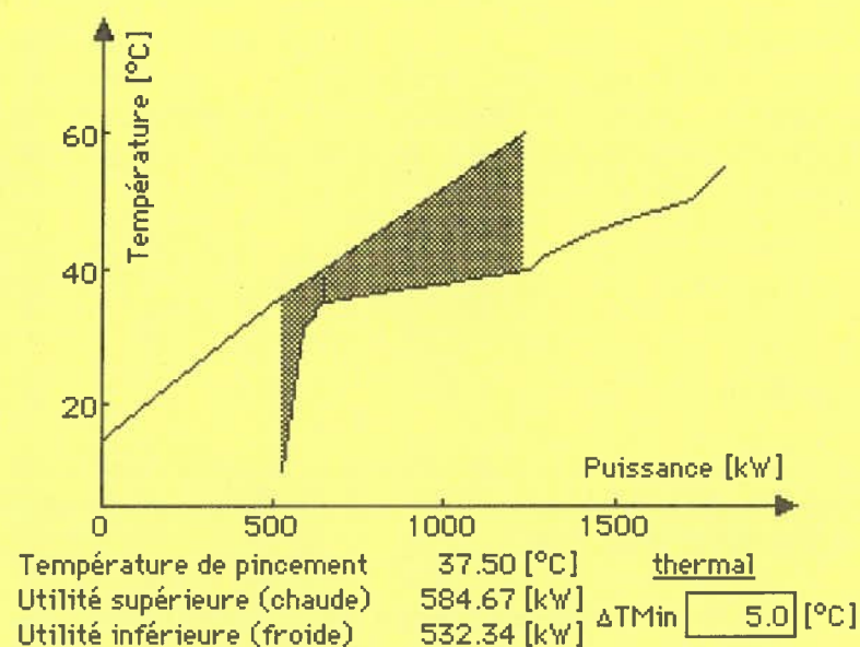
Figure 10a: Composites correspondant au cahier des charges de l'établissement thermal.
