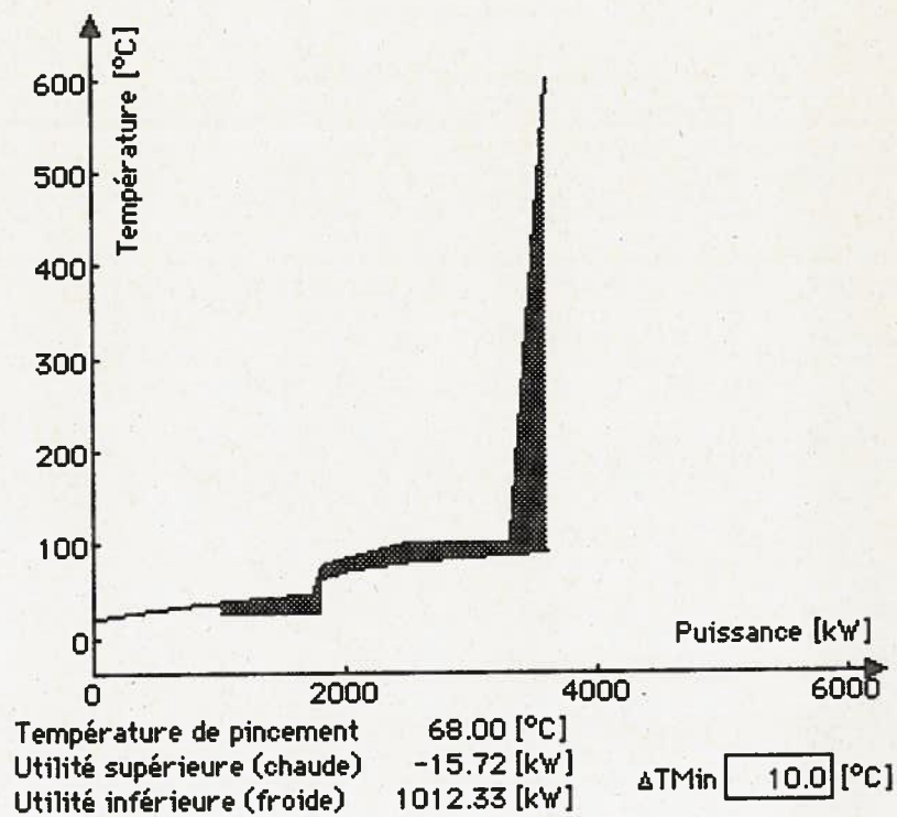
Figure 41b: Composites avec une pompe à chaleur à moteur thermique.
