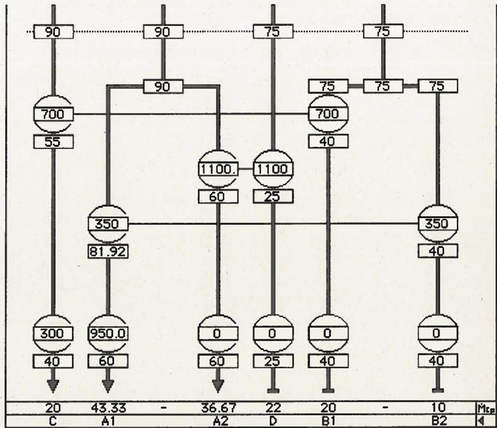
Figure 15a: Première alternative de réseau à consommation d'énergie minimum pour la zone source.
