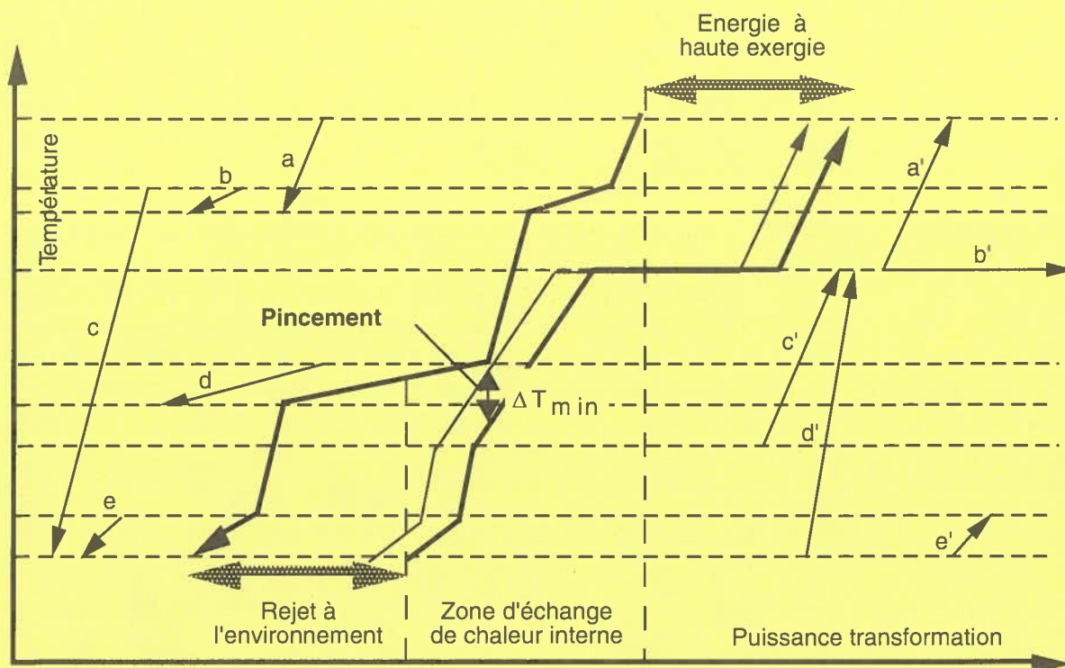
Figure 3: Vecteurs flux et courbes composites dans un diagramme Température – Puissance-transformation.
