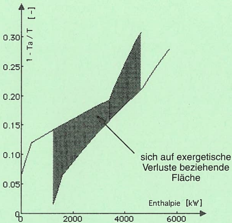
Abb. 6: Exergetische Verluste der internen Wärmeübertragung.
