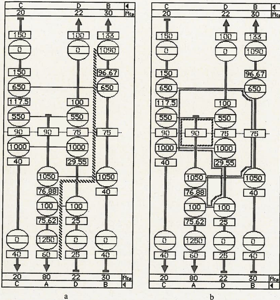
Figure 18: Nouveau réseau sans dédoublement au niveau de la source.
