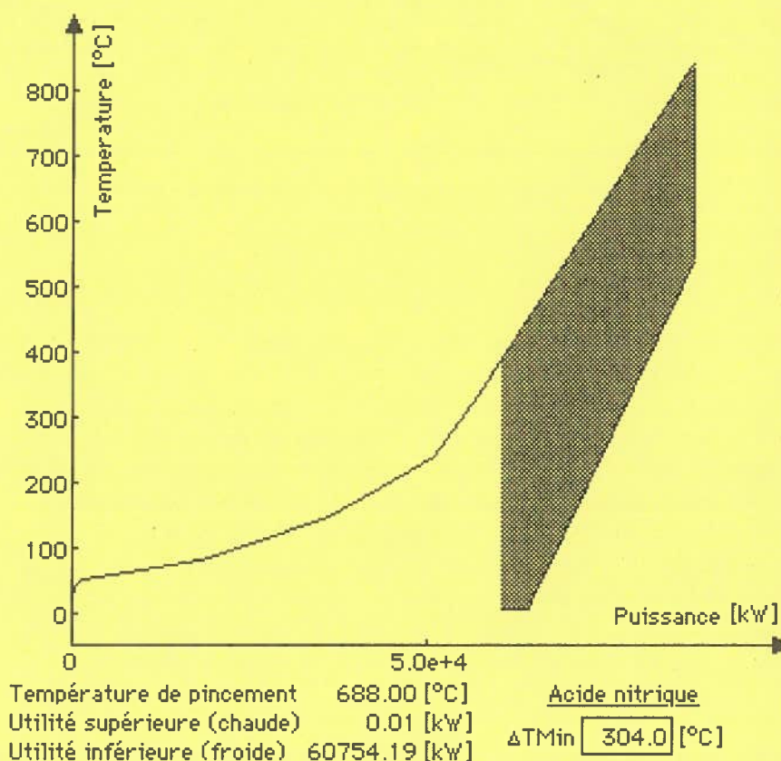
Figure 4a: Composites de l'installation d'acide nitrique seule.
