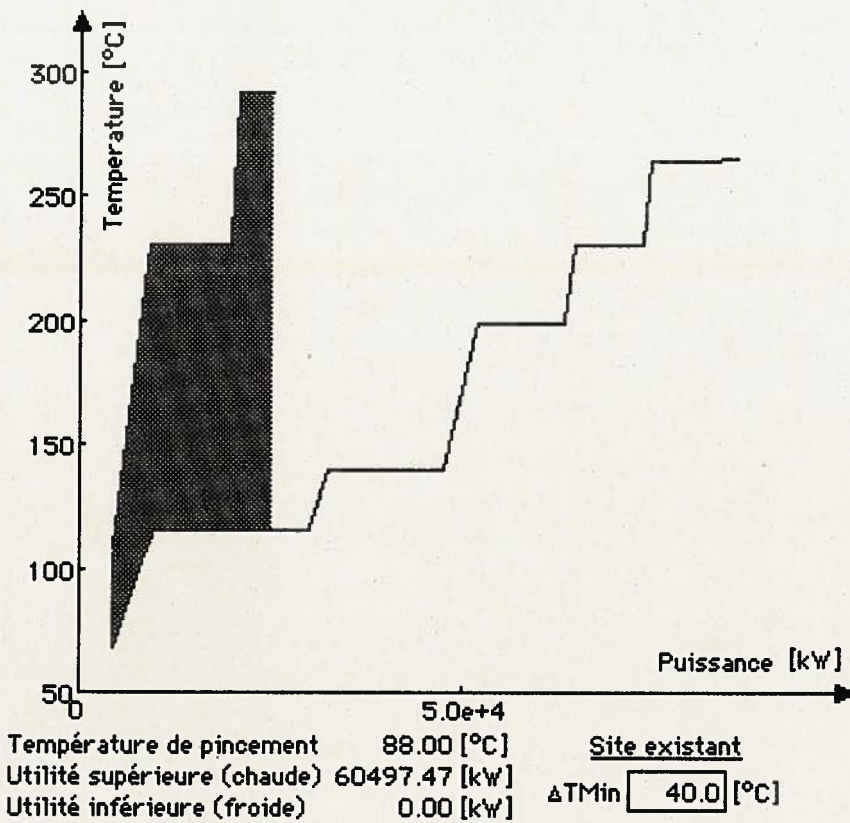
Figure 12b: Composites du site existant.
