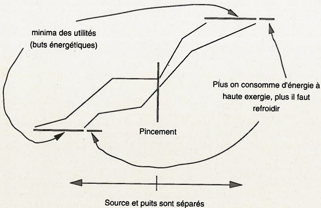
Figure 6: Influence du \Delta T_{min} sur les minima de consommations énergétiques.
