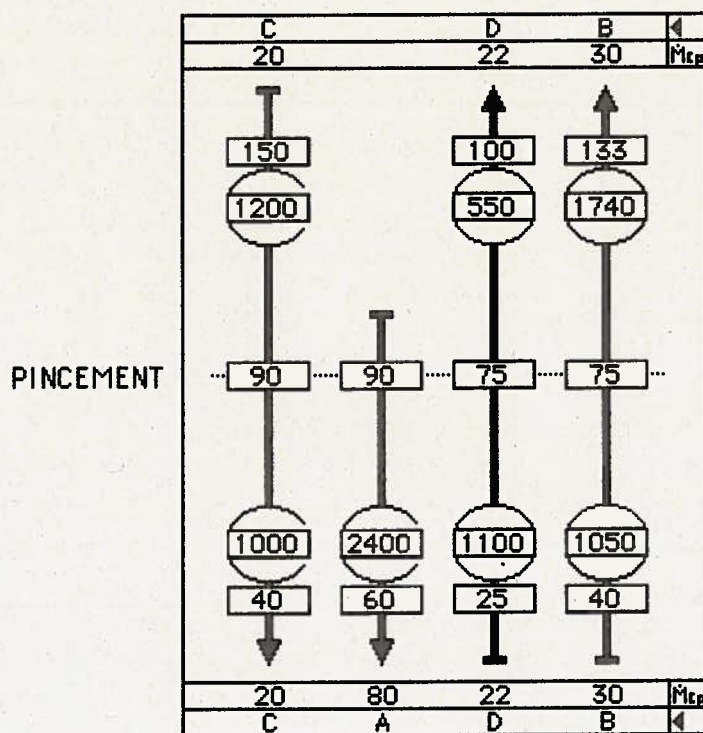
Figure 13: Diagramme de représentation des flux et échangeurs d'utilités.
