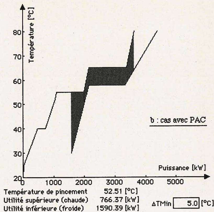
Figure 38: Intégration d'une pompe à chaleur à cycle ouvert dans un procédé.
