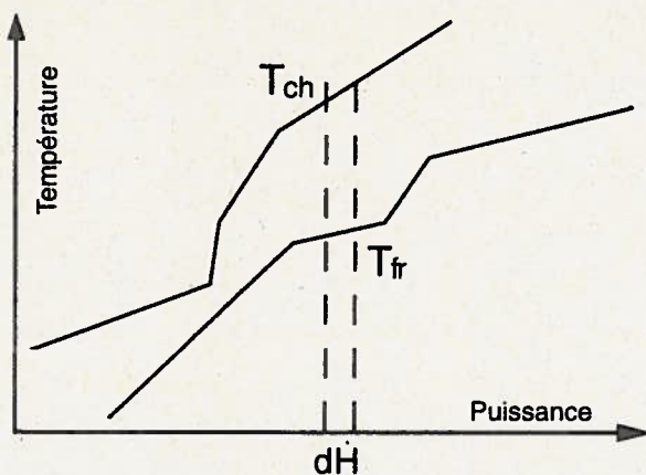
Figure 25: Méthode de calcul de la surface totale d'échangeurs.
