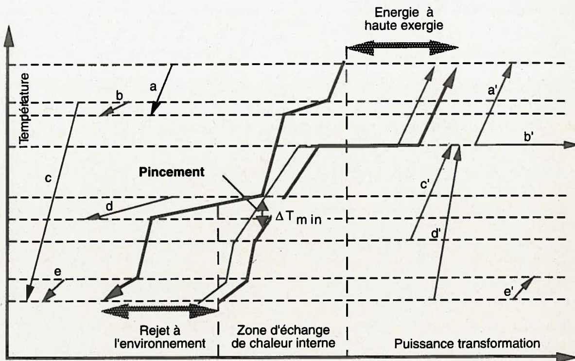
Figure 5: Vecteurs flux et courbes composites dans un diagramme Température - Puissance-transformation.
