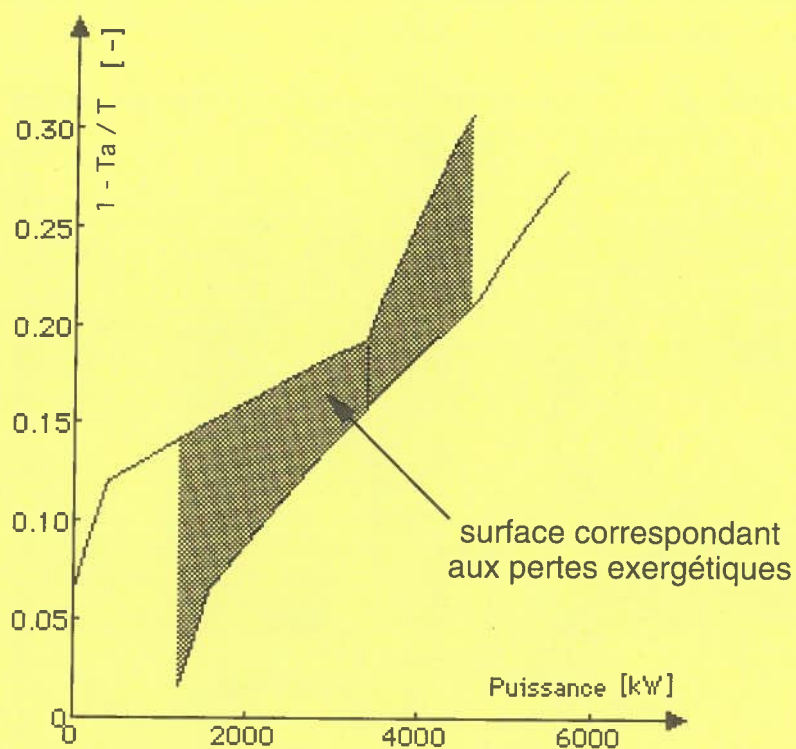
Figure 6: Représentation des pertes exergétiques de transfert de chaleur interne (voir aussi réf. 10).
