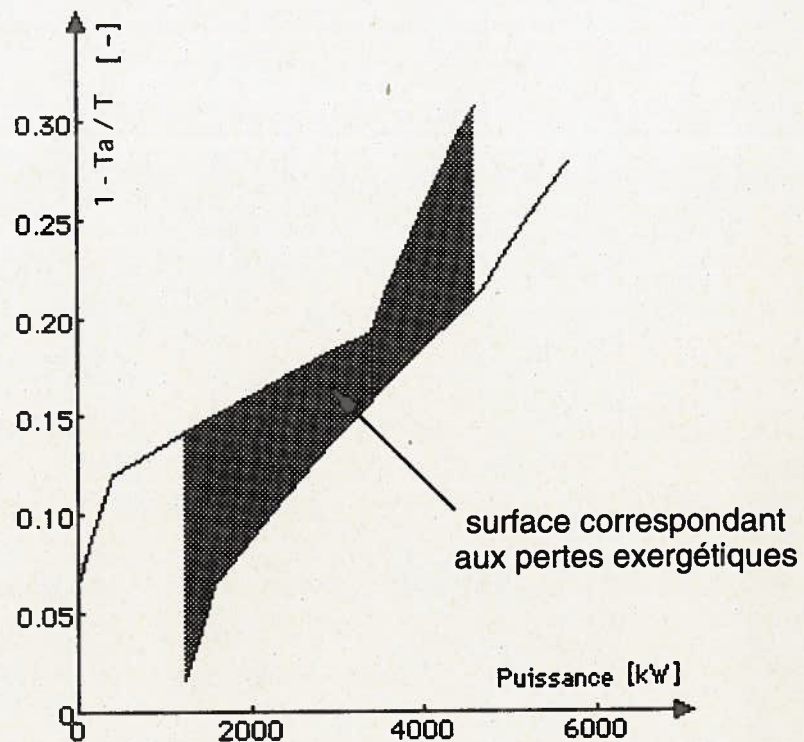
Figure 10: Représentation des pertes exergétiques de transfert de chaleur interne.
