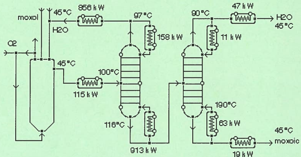
Abb. 7: Vereinfachtes Schema der Produktion von Methoxyessigsäure.
