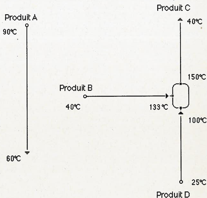
Figure 4b: Schéma d'écoulement simplifié de l'exemple du procédé de la figure 4a.
