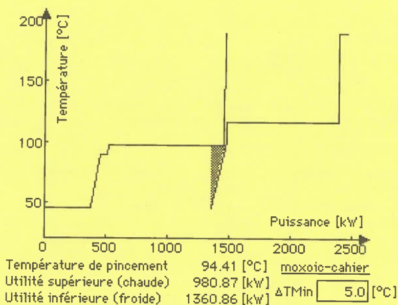
Figure 8a: Composites du procédé initial de fabrication de l'acide méthoxyacétique.
