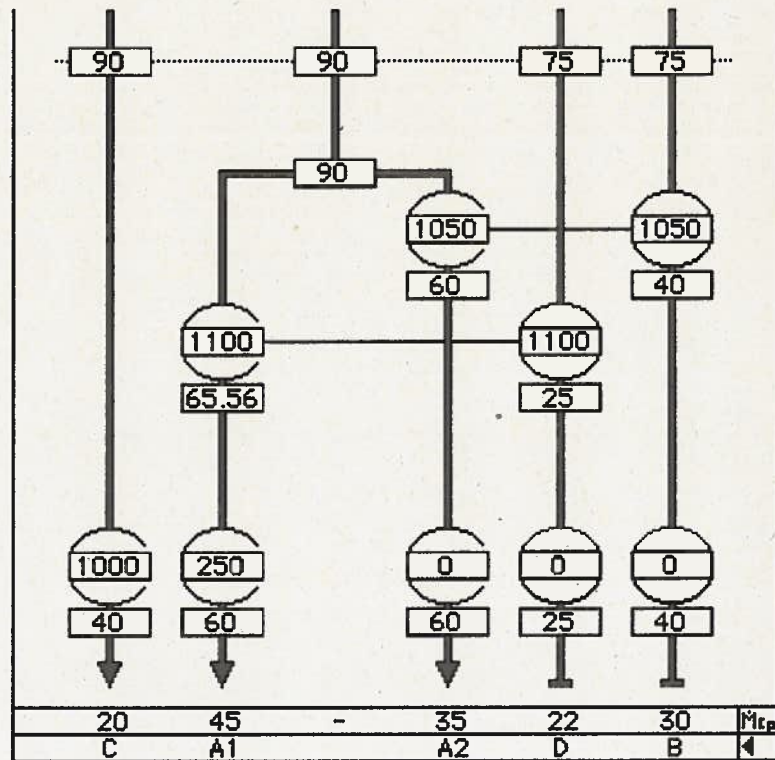
Figure 15b: Deuxième alternative de réseau à consommation d'énergie minimum pour la zone source.
