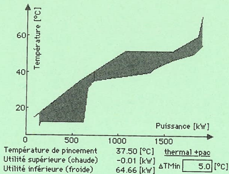
Abb.10b: Composite Curves des ausschließlich mit einer Wärmepumpe beheizten Thermalbades.
