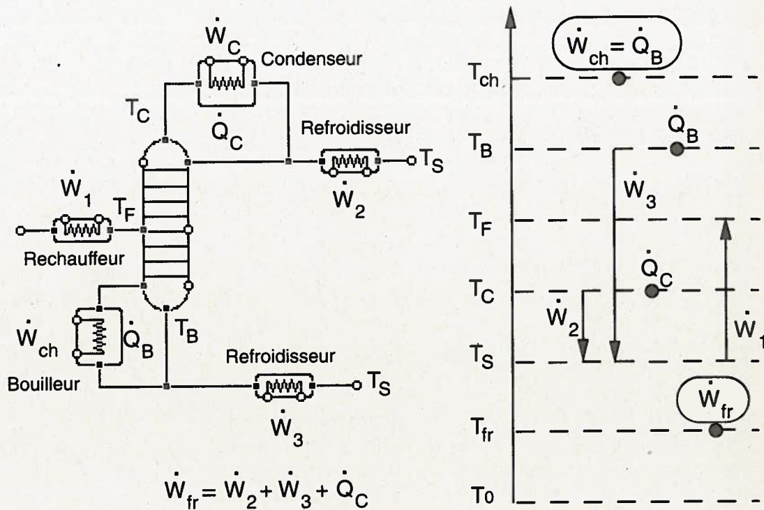
Figure 42: Intégration de colonnes de distillation.
