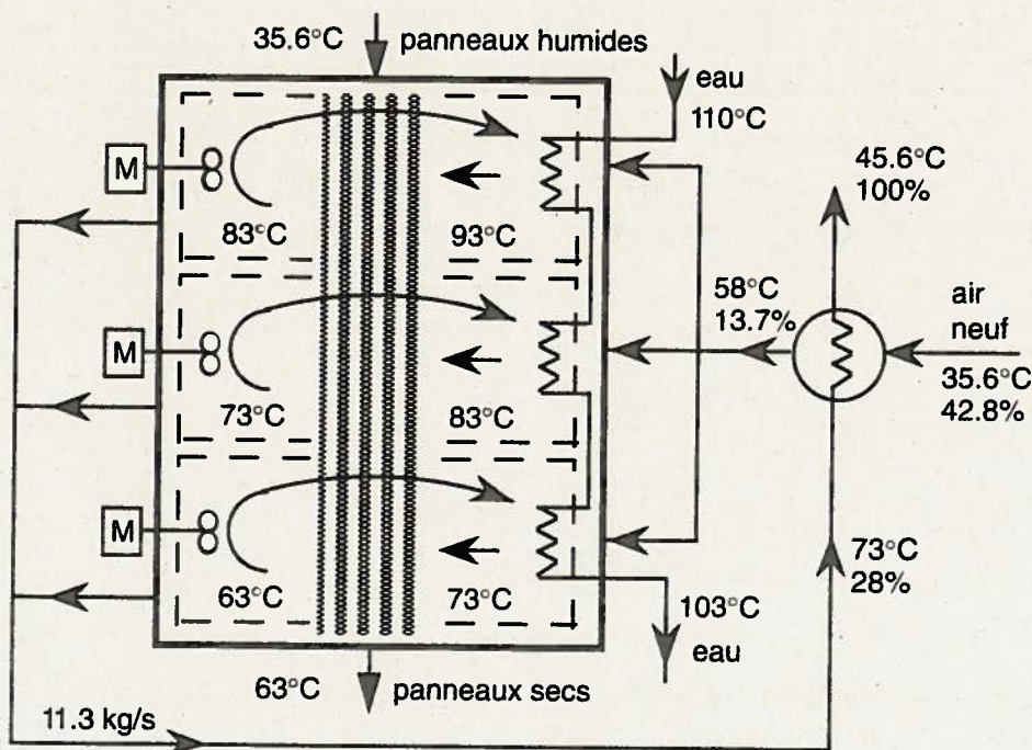
Figure 40: Procédé de séchage de panneaux de plâtre.
