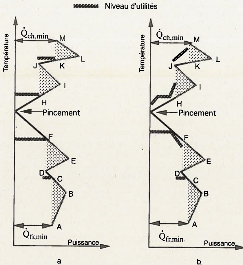
Figure 29: Détermination des niveaux d'utilités minimum (puits), resp. maximum (source).
