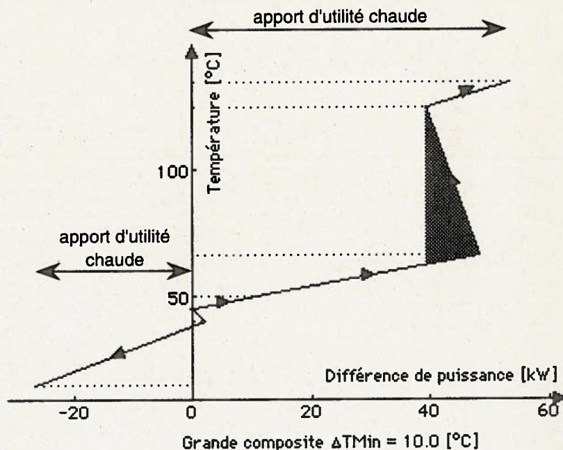
Figure 30a: Grande composite relative au cas limite de la table 2 avec \Delta T_{min} = 10^\circ C .
