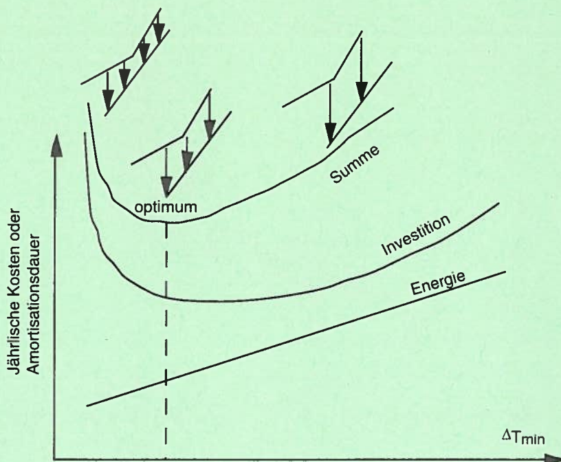
Abb. 5: Entwicklung der verschiedenen Kosten in Abhängigkeit von \Delta T_{min} .
