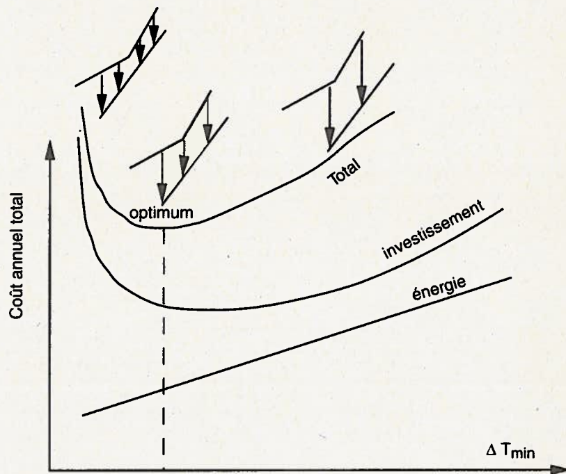
Figure 26: Evolution des différents coûts en fonction du \Delta T_{min} .
