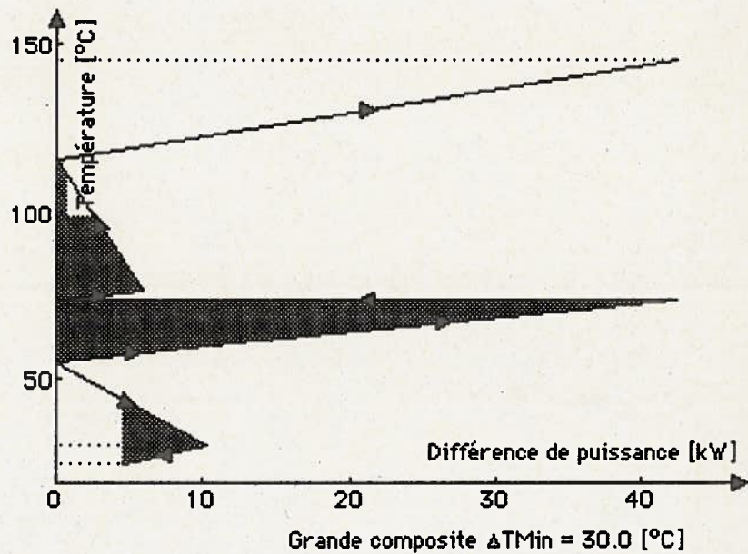
Figure 32: Introduction d'un apport de vapeur à 88.5°C (73.5°C dans le diagramme de la grande composite) dans le cas de la figure 30c. Apparition de deux pincements externes.
