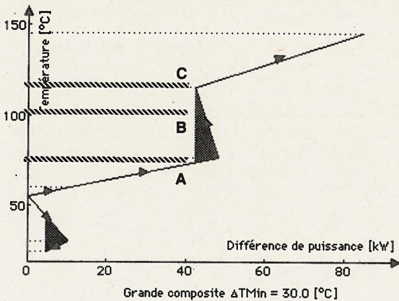
Figure 30c: Grande composite relative au cas limite de la table 2 avec \Delta T_{\min} = 30^{\circ}\text{C} .
