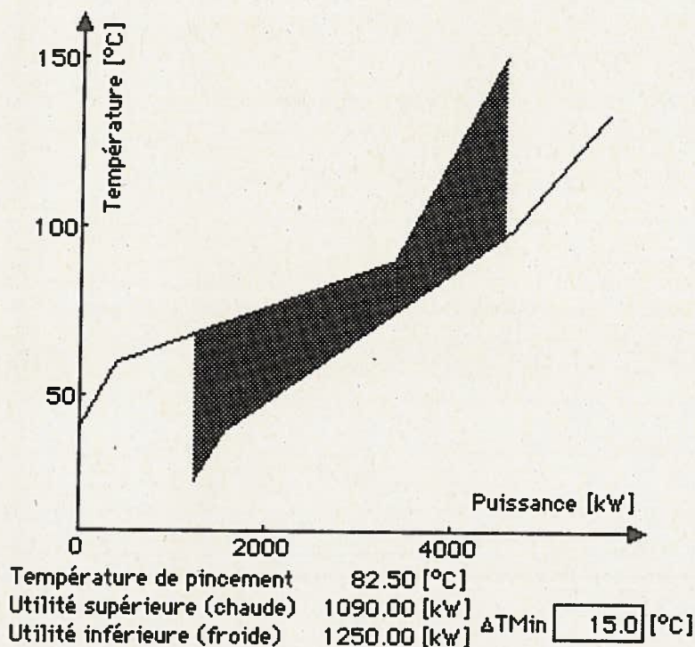
Figure 8: Résultats obtenus par le programme PINCHY (réf. 8).
