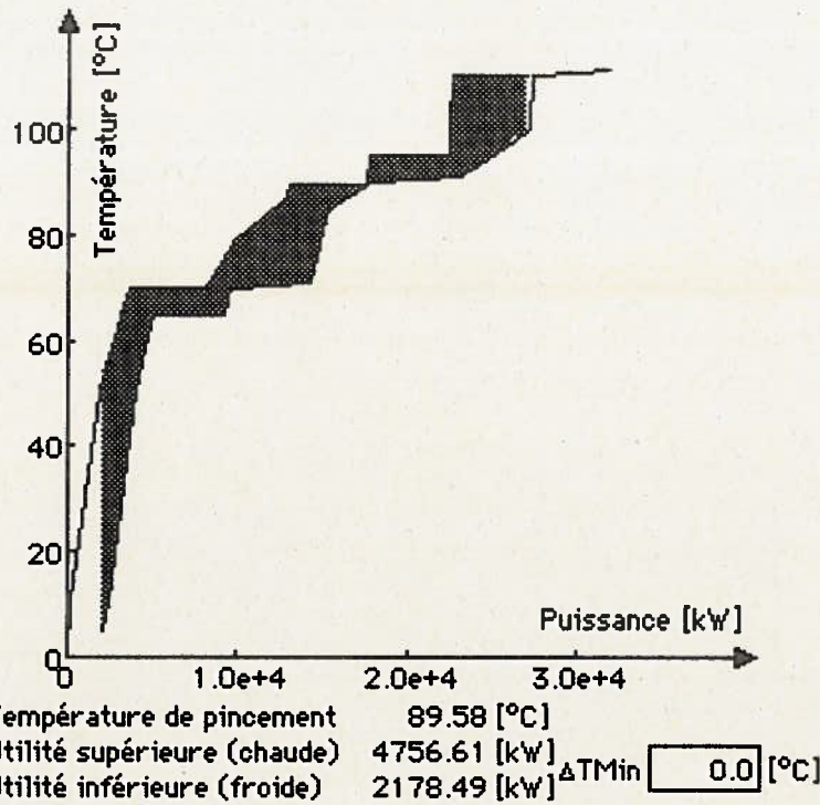
Figure 39d: Même procédé et même cycle de pompe à chaleur fermée mais en alimentant l'évaporateur qu'avec les flux de la zone source (pas de déplacement de la température de pincement).
