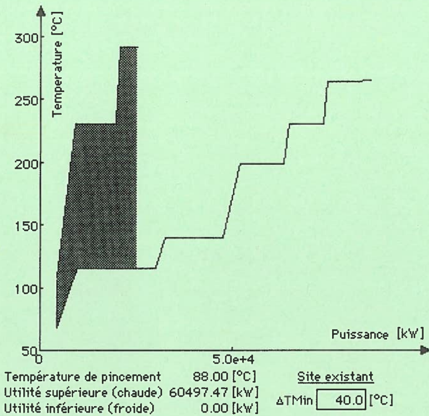
Abb. 4b: Composite Curves der existierenden Anlage.
