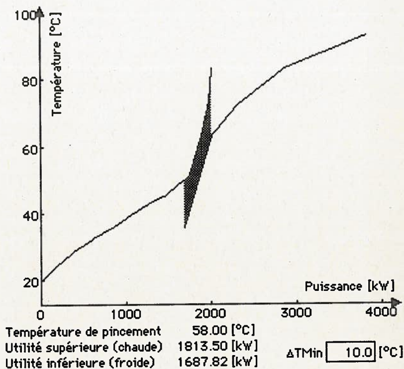
Figure 41a: Composites du procédé de séchage de panneaux de plâtre initial.
