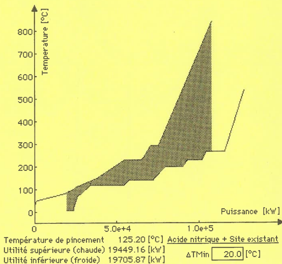
Figure 4c: Composites du site + acide nitrique.
