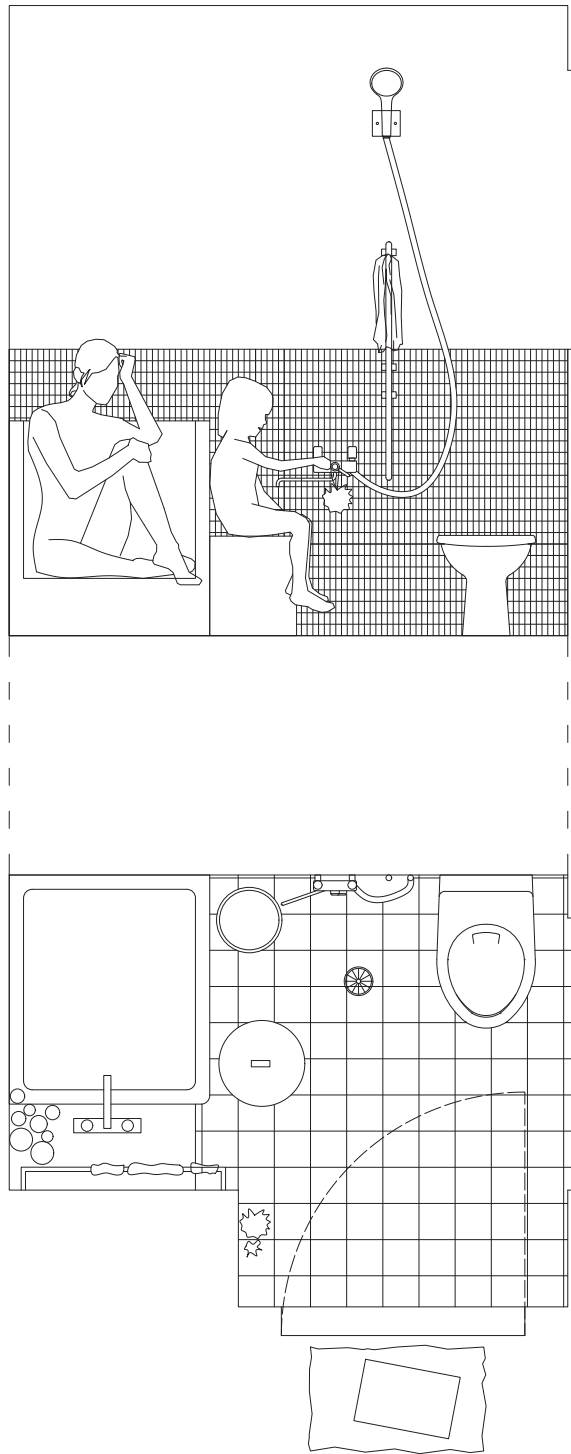
Figure49: (Une Affaire de f.) Mise en plan et en coupe de la salle de bain
