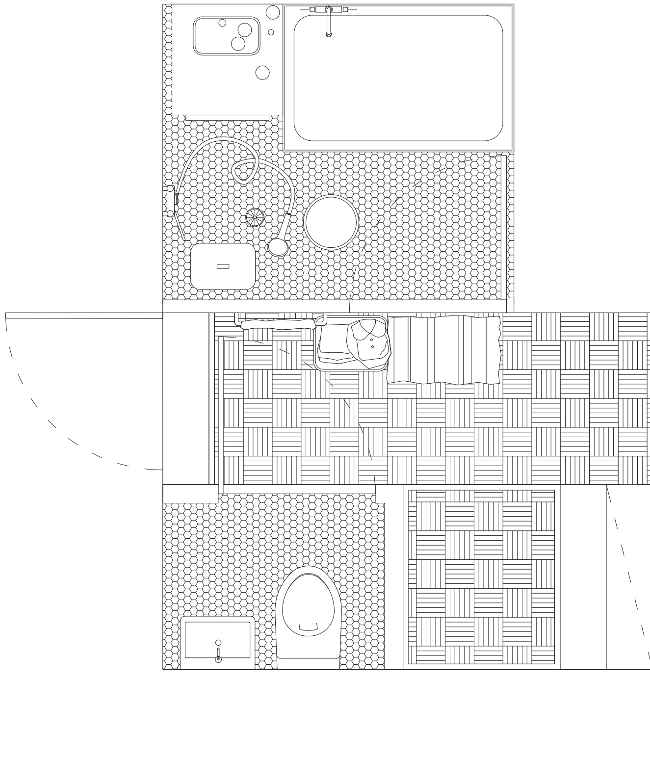
Figure46: (Air Doll) Mise en dessin du plan de la salle de bain et WC 1:20
