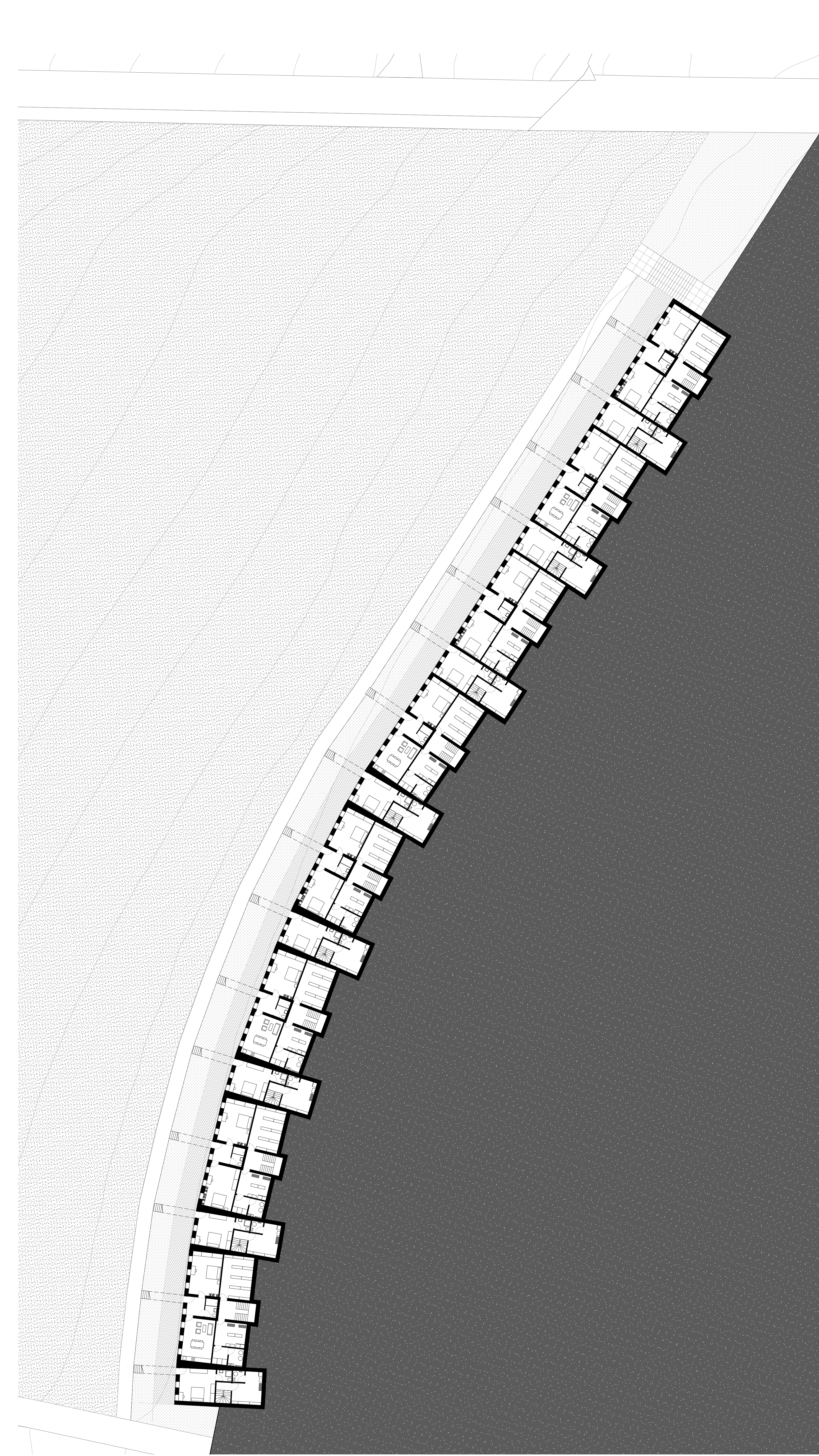
Rez-de-chaussée semi-enterré - Plan 1:250
