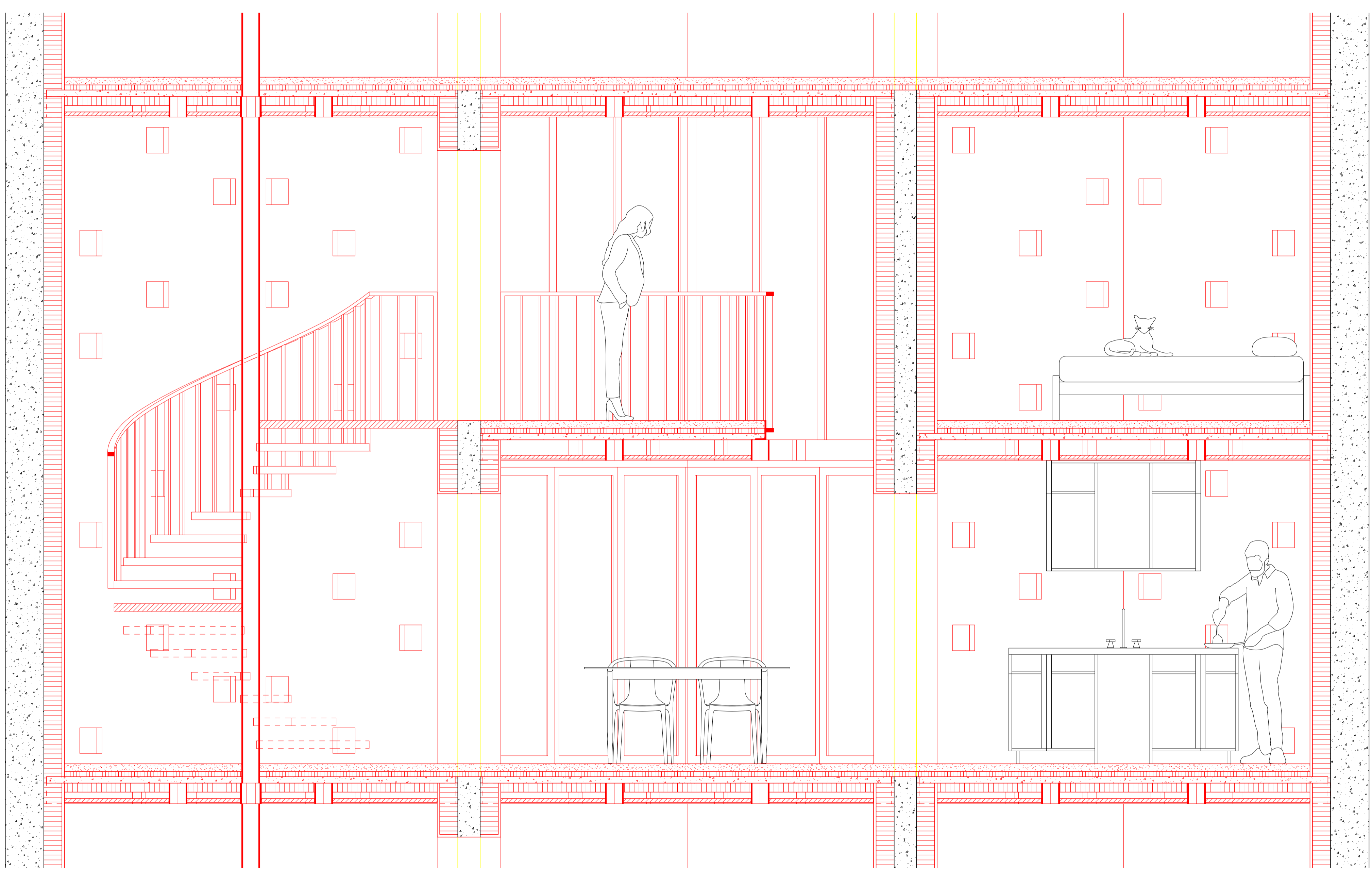
Coupe type 1:20
