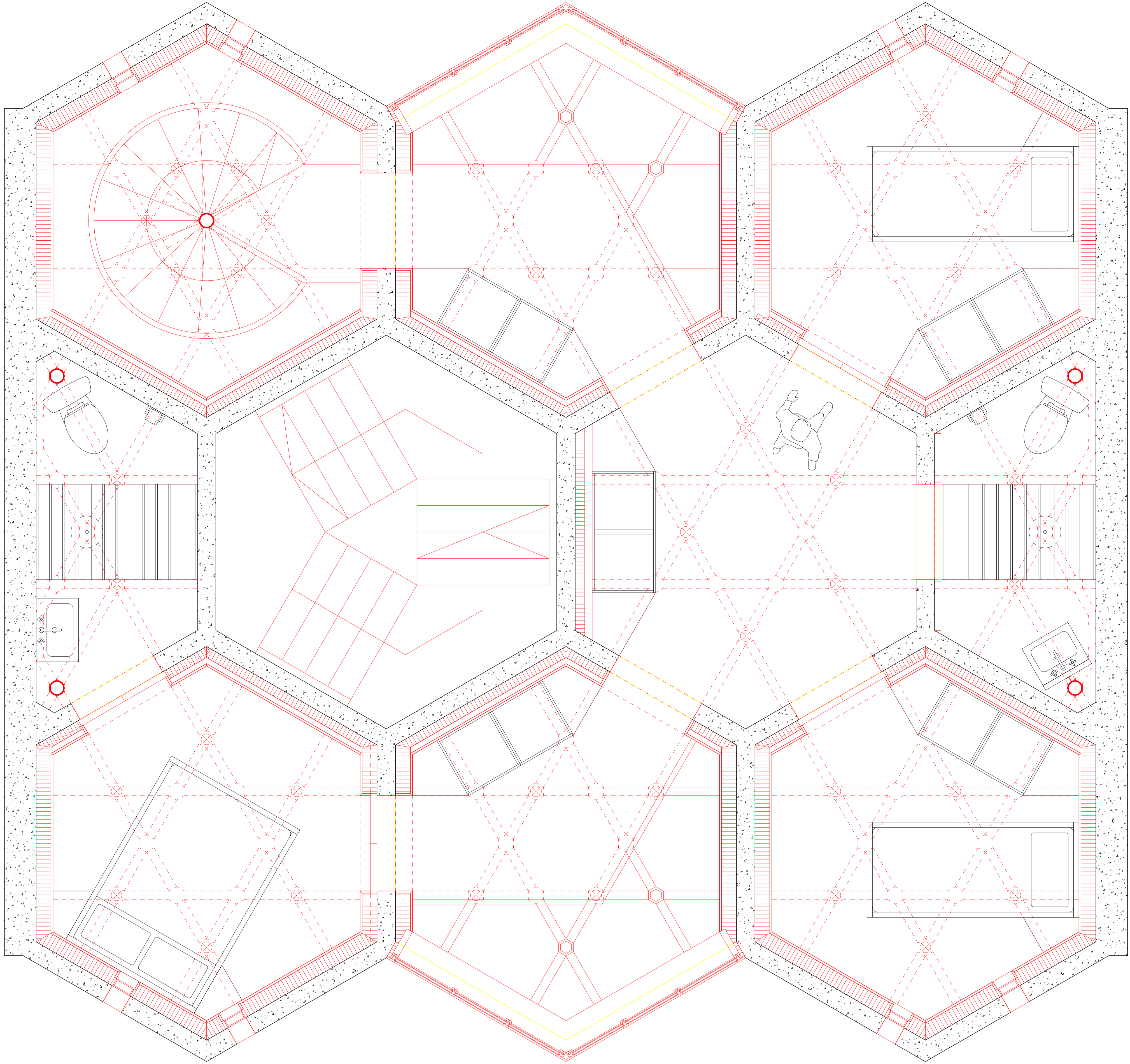
Etage inférieur type 1:20
