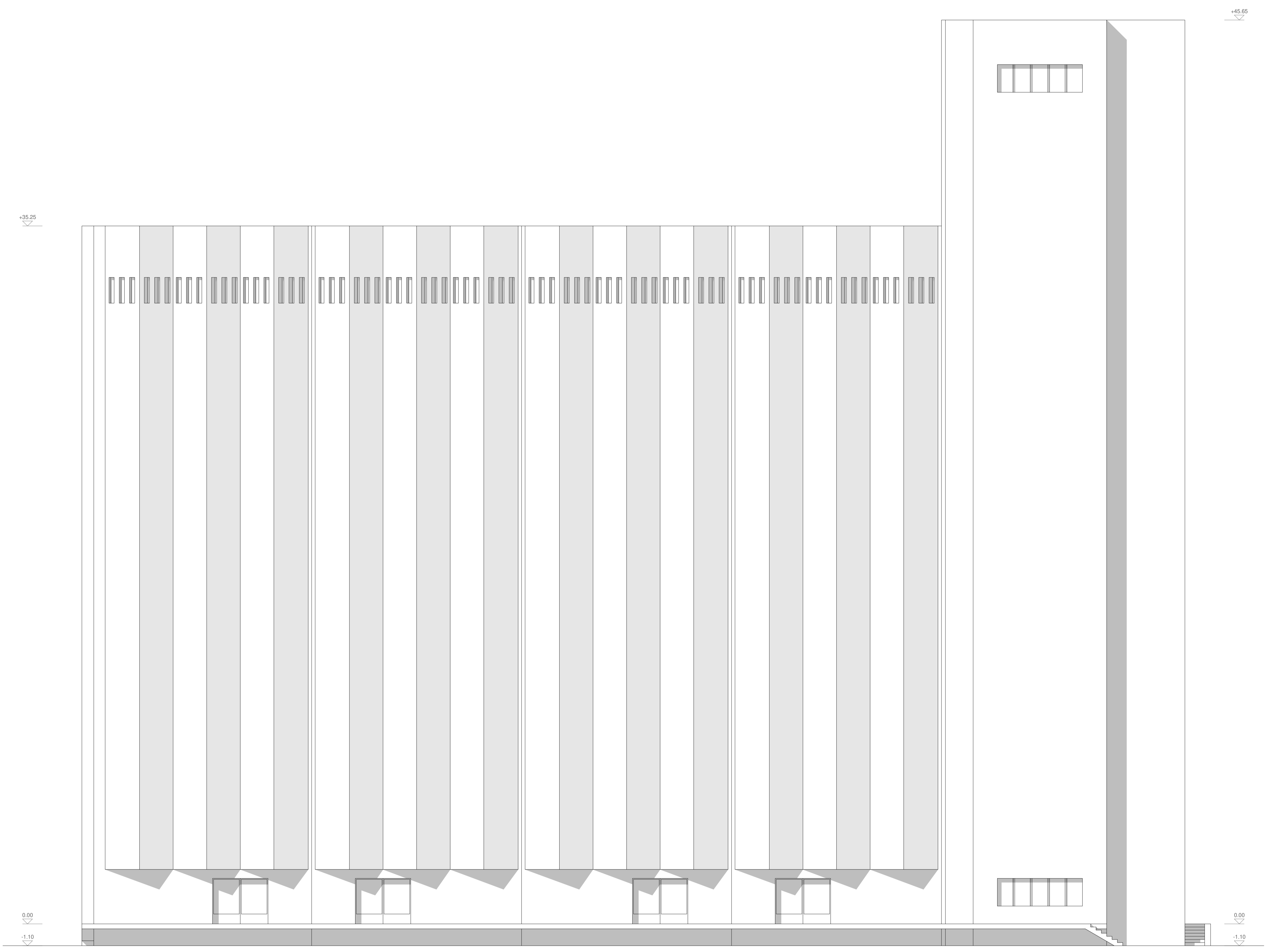
Façade sud existante 1:100
