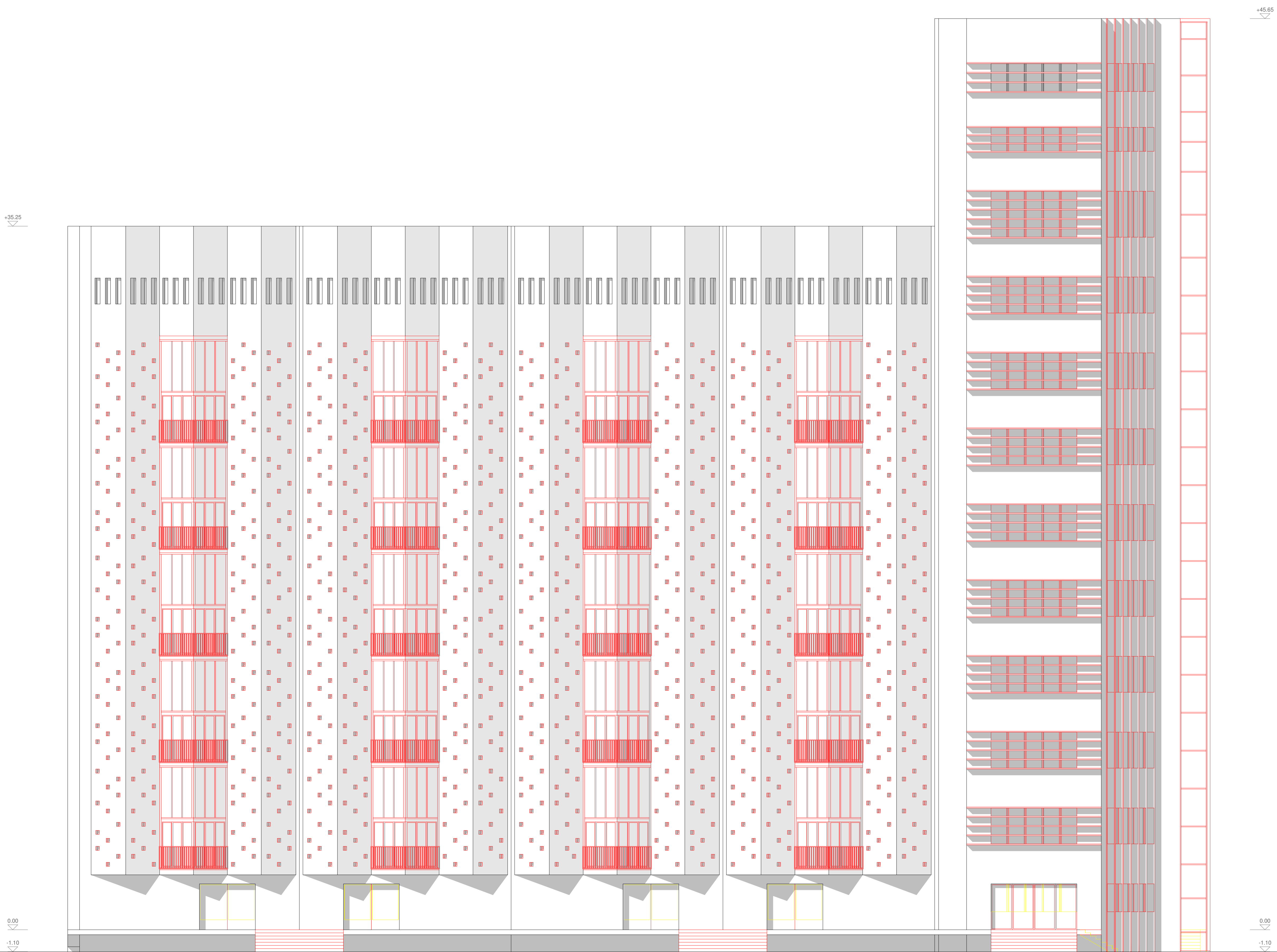
Façade sud projetée 1:100
