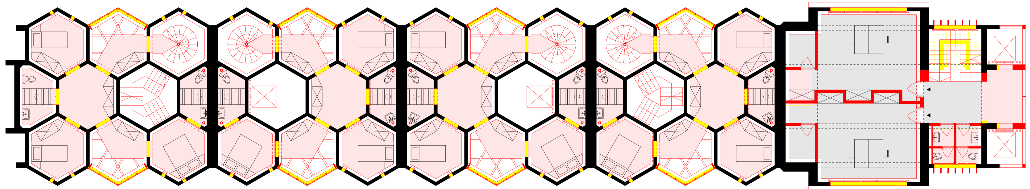
Plan d'étage supérieur type projeté 1:100
