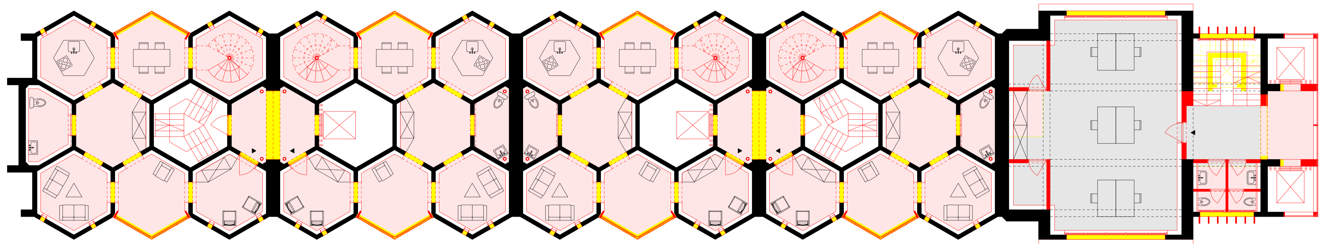
Plan d'étage inférieur type projeté 1:100
