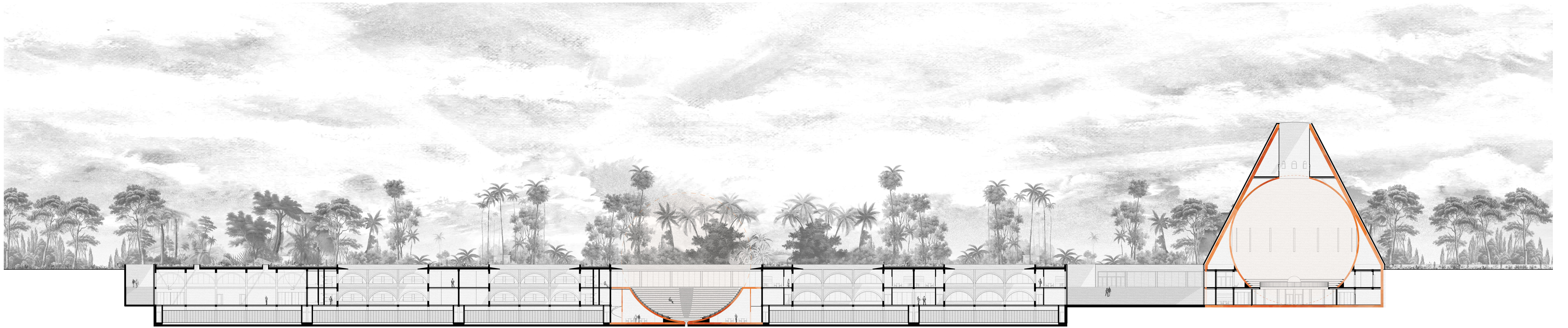
a. La coupe longitudinale sur les patios au sud
