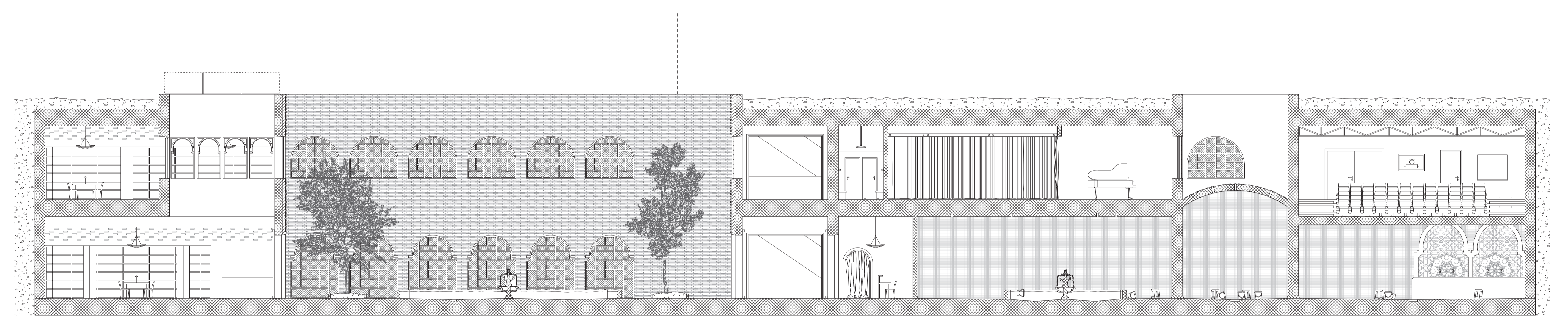
Coupe AA'
