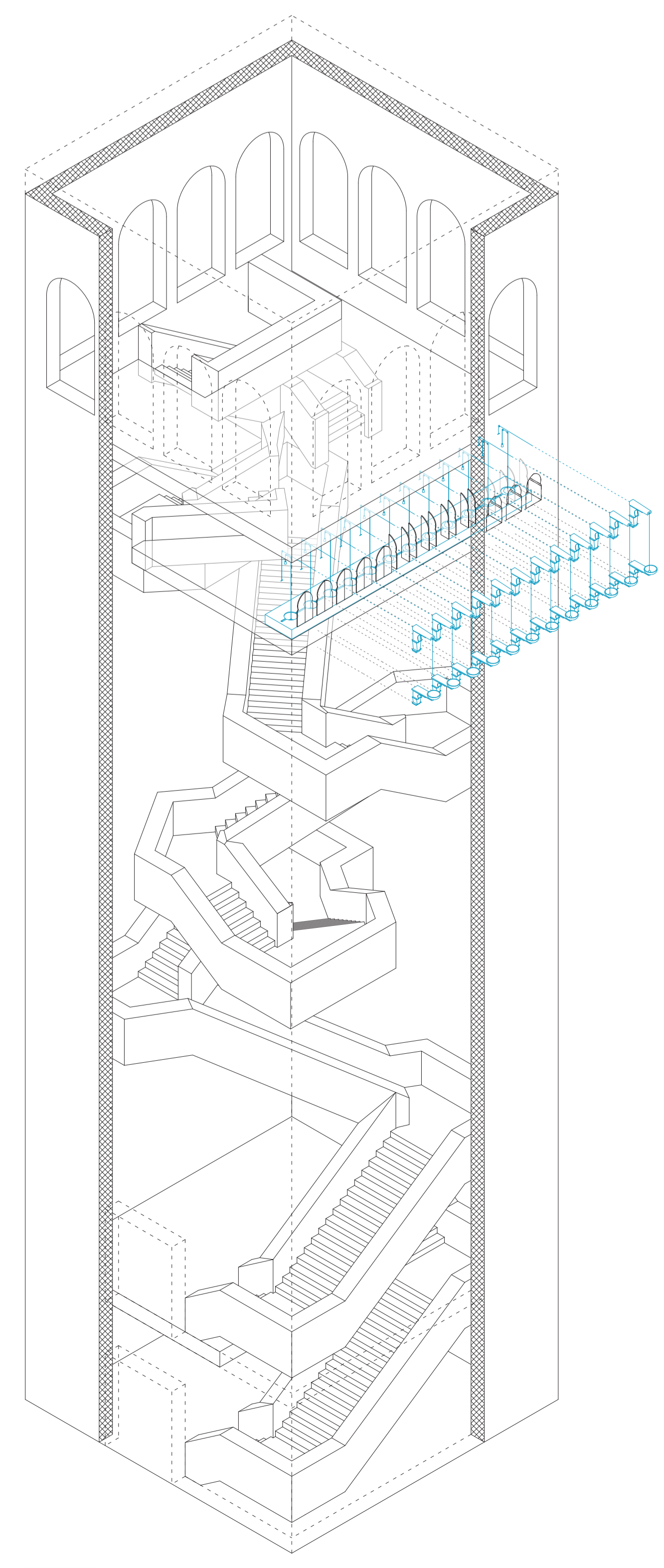
Axonométrie de la tour et de son horloge hydraulique
