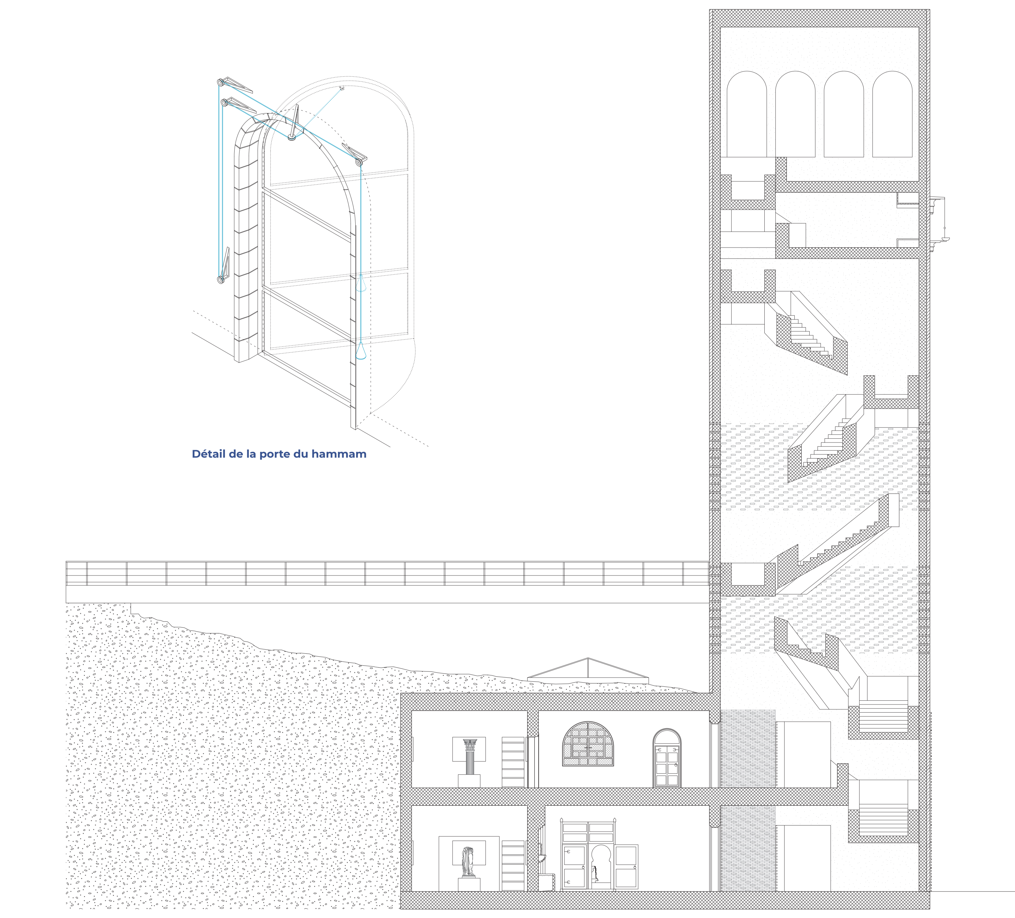
Coupe BB'
