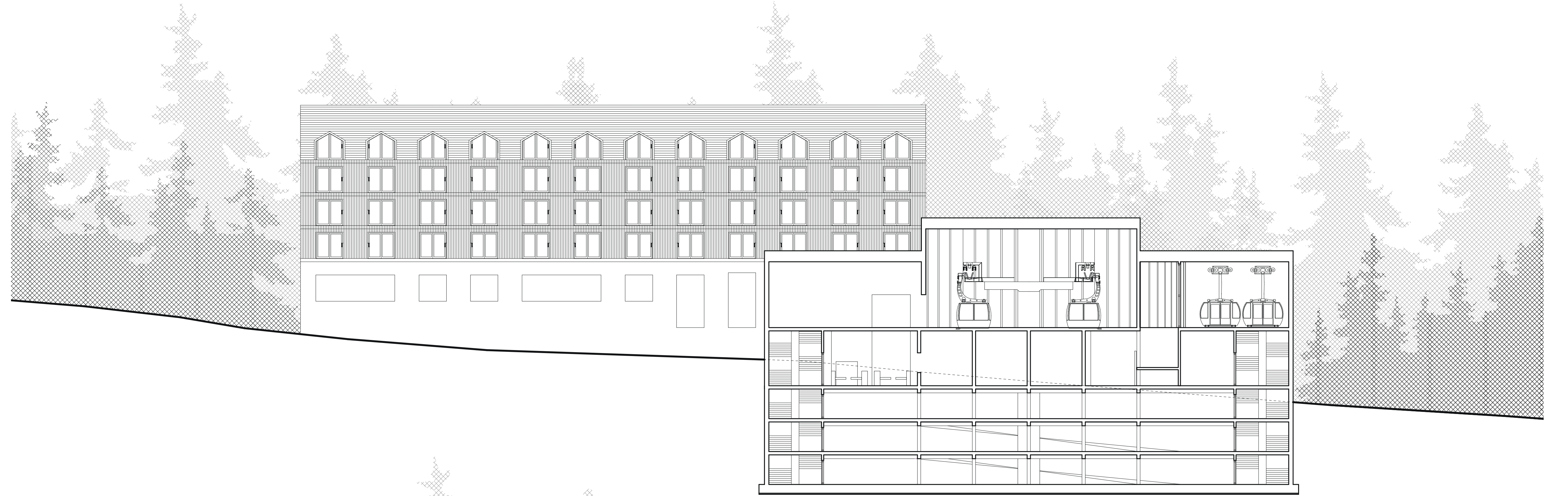
Coupe AA_ 1: 200
