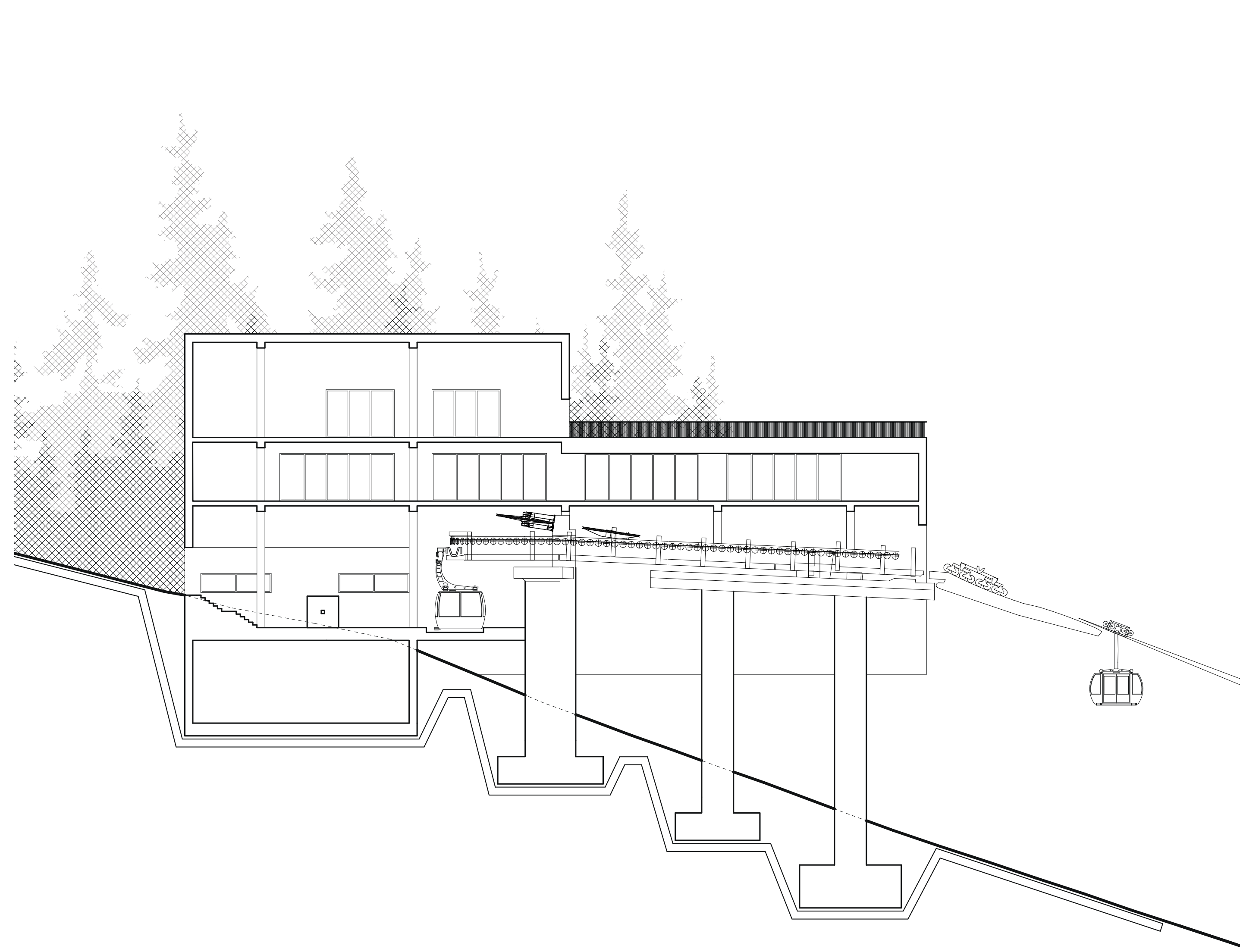
Coupe CC_ 1: 200
