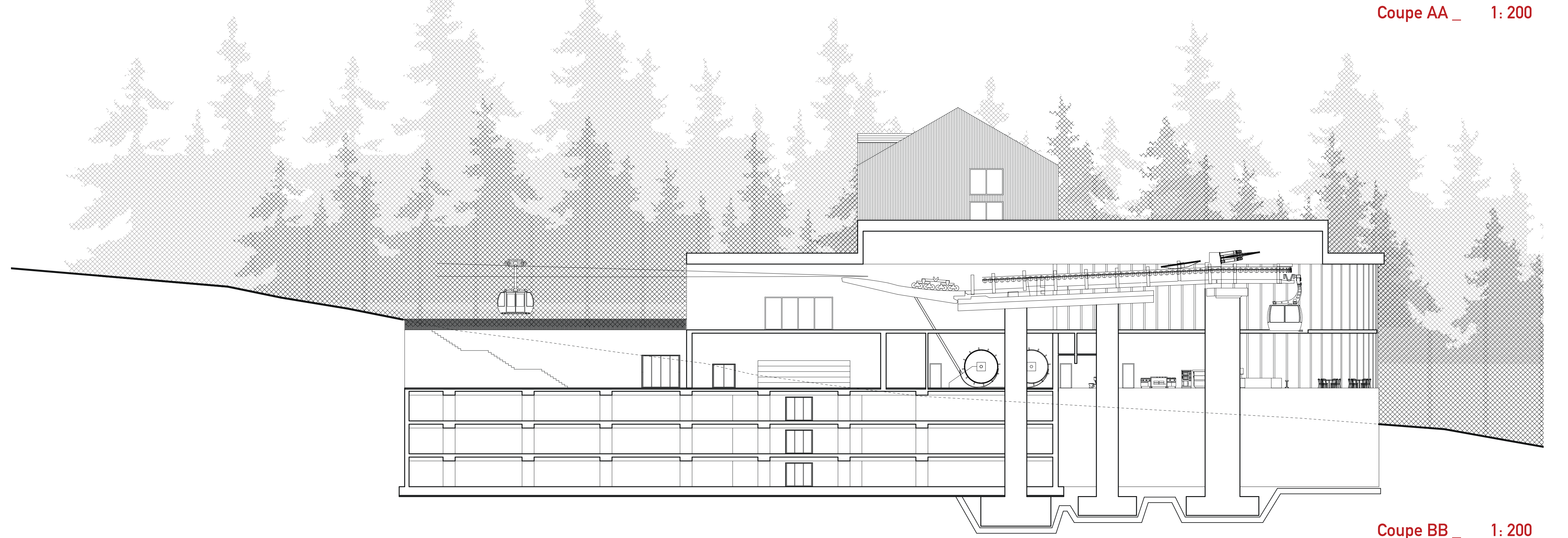
Coupe BB_ 1: 200
