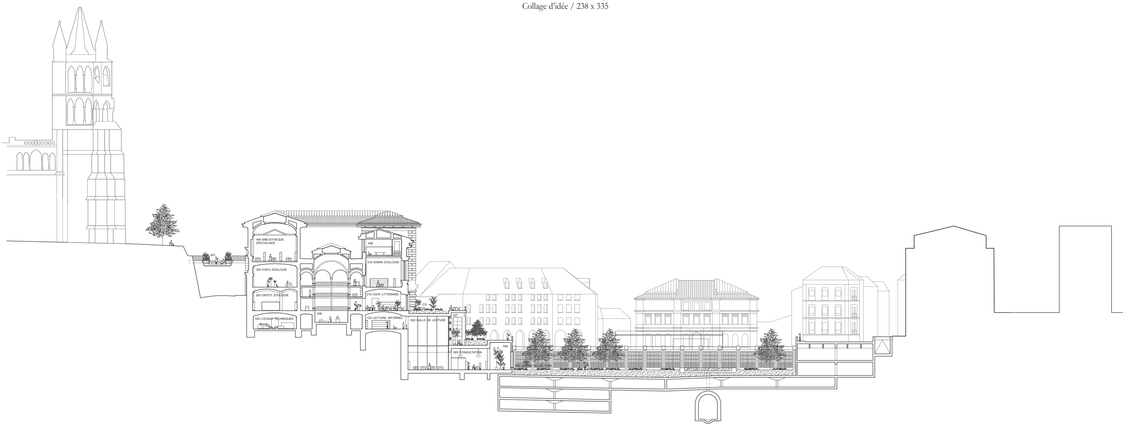
5 Coupe transversale sud 1:500
