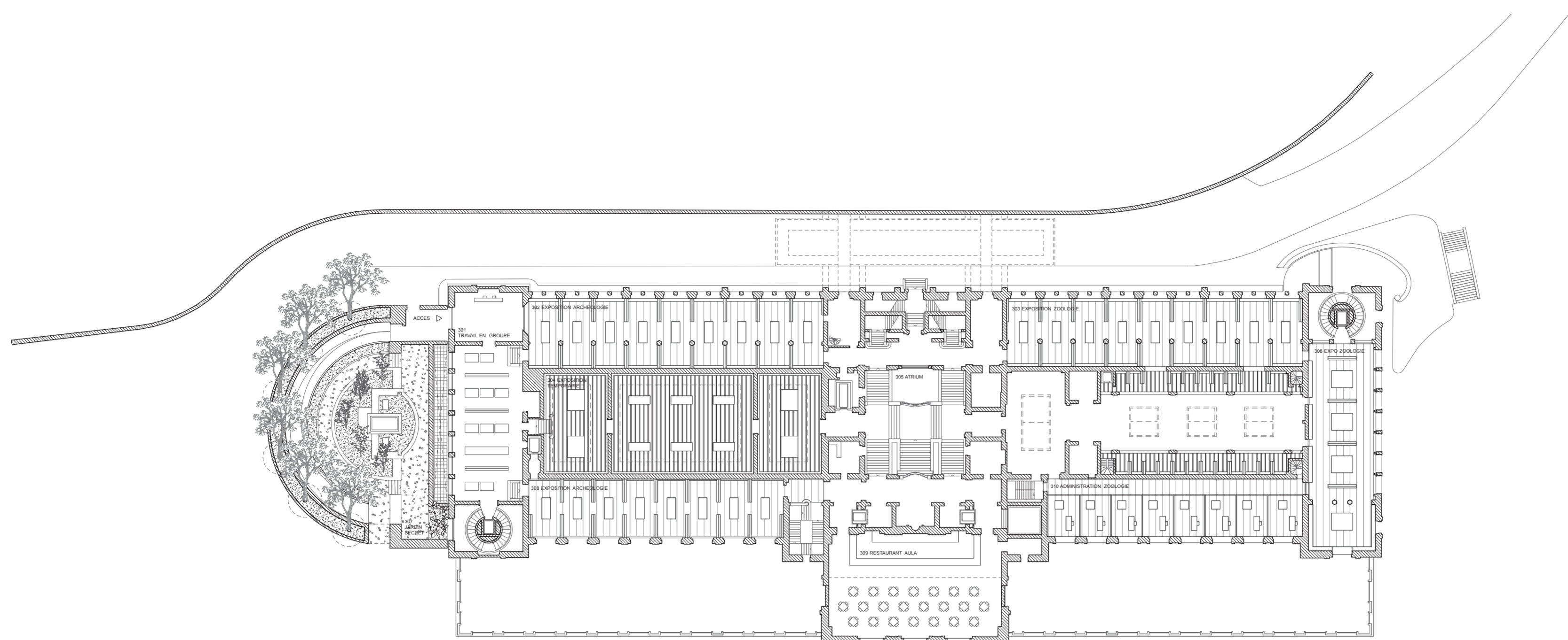
3 Plan niveau 3 1:500
