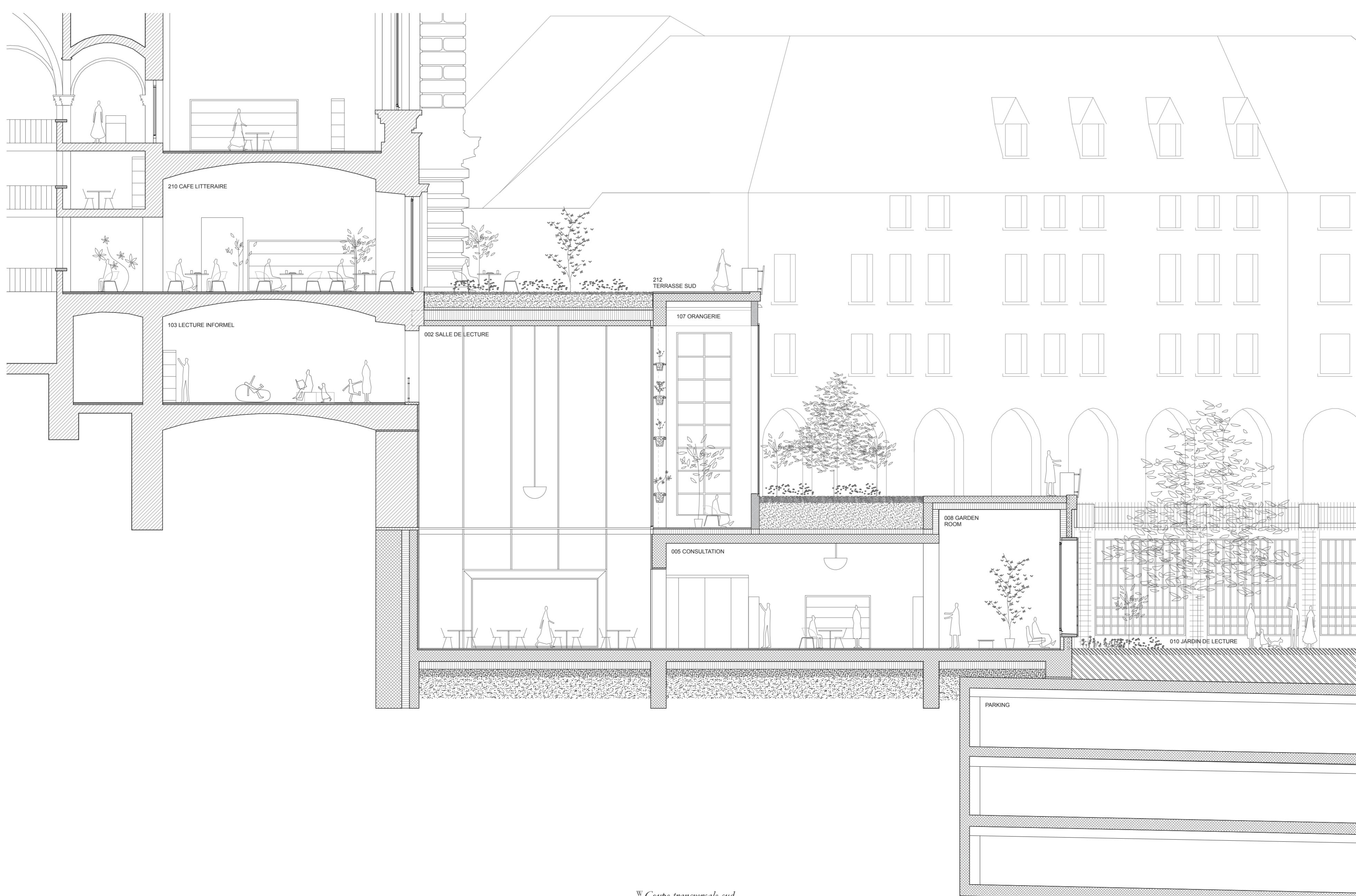
6 Coupe transversale sud 1:100
