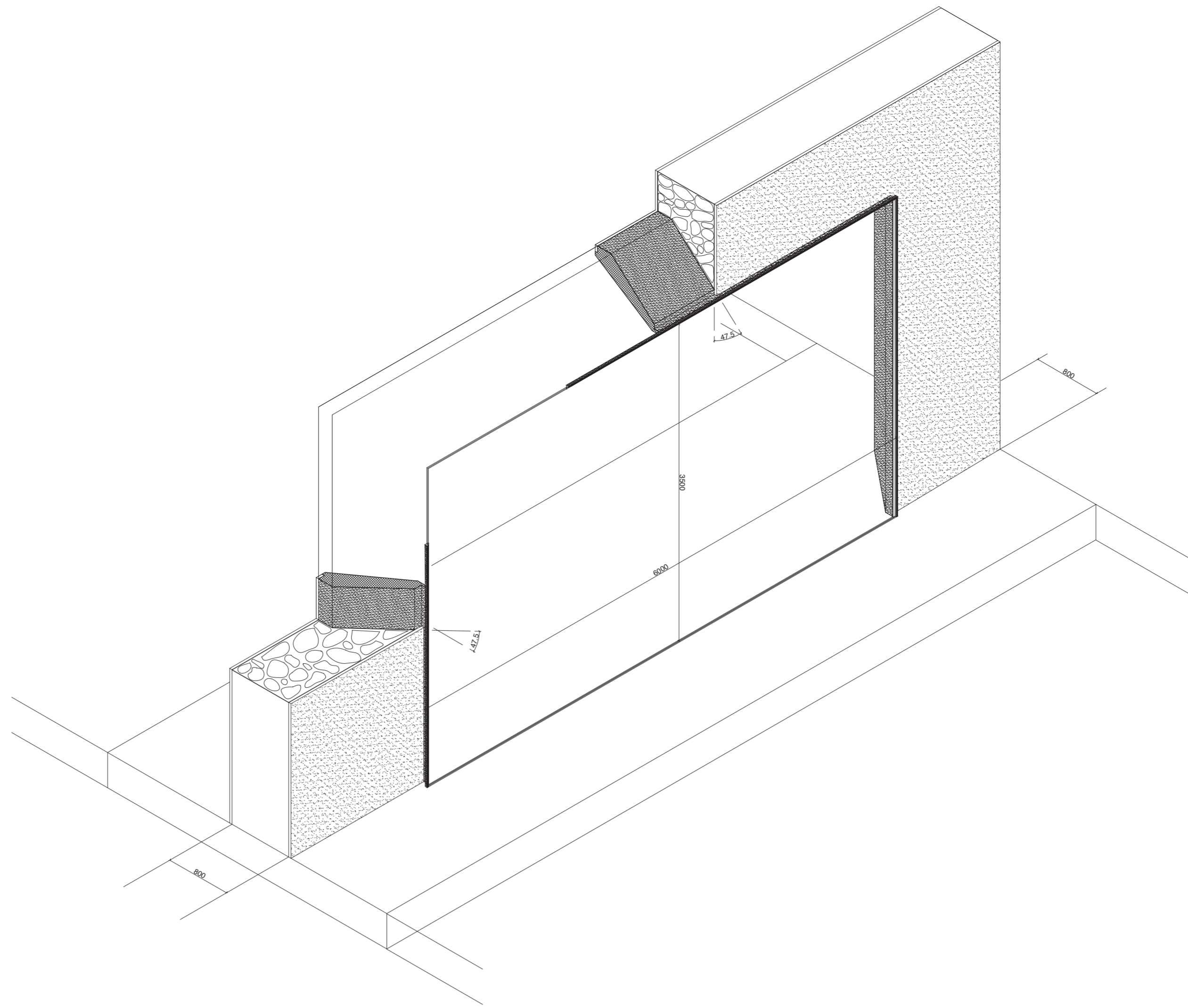
1 Intervention sur existant Axonométrie détail
