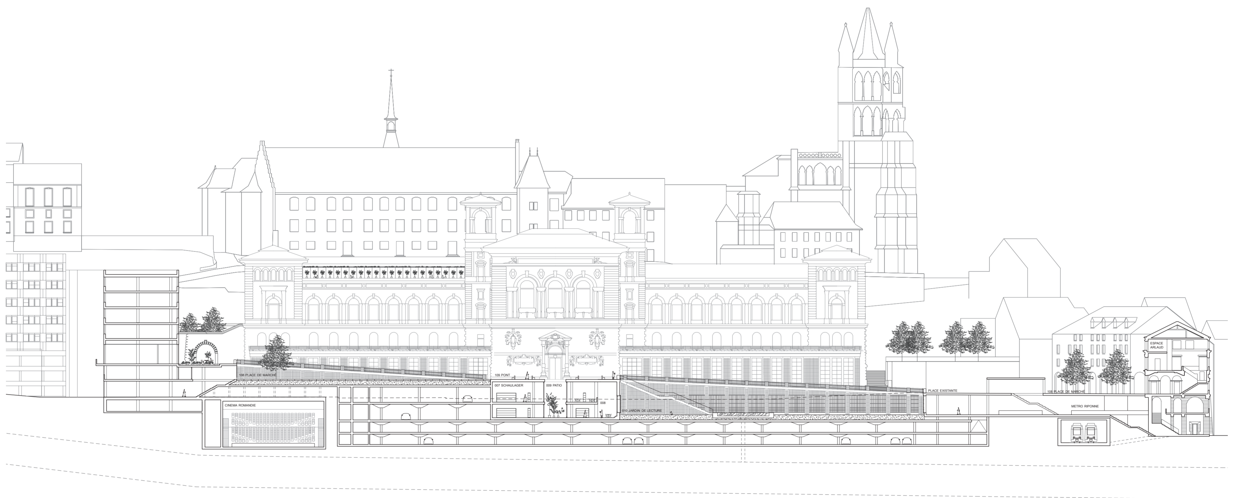
6 Coupe longitudinale nord-sud NS 1:500
