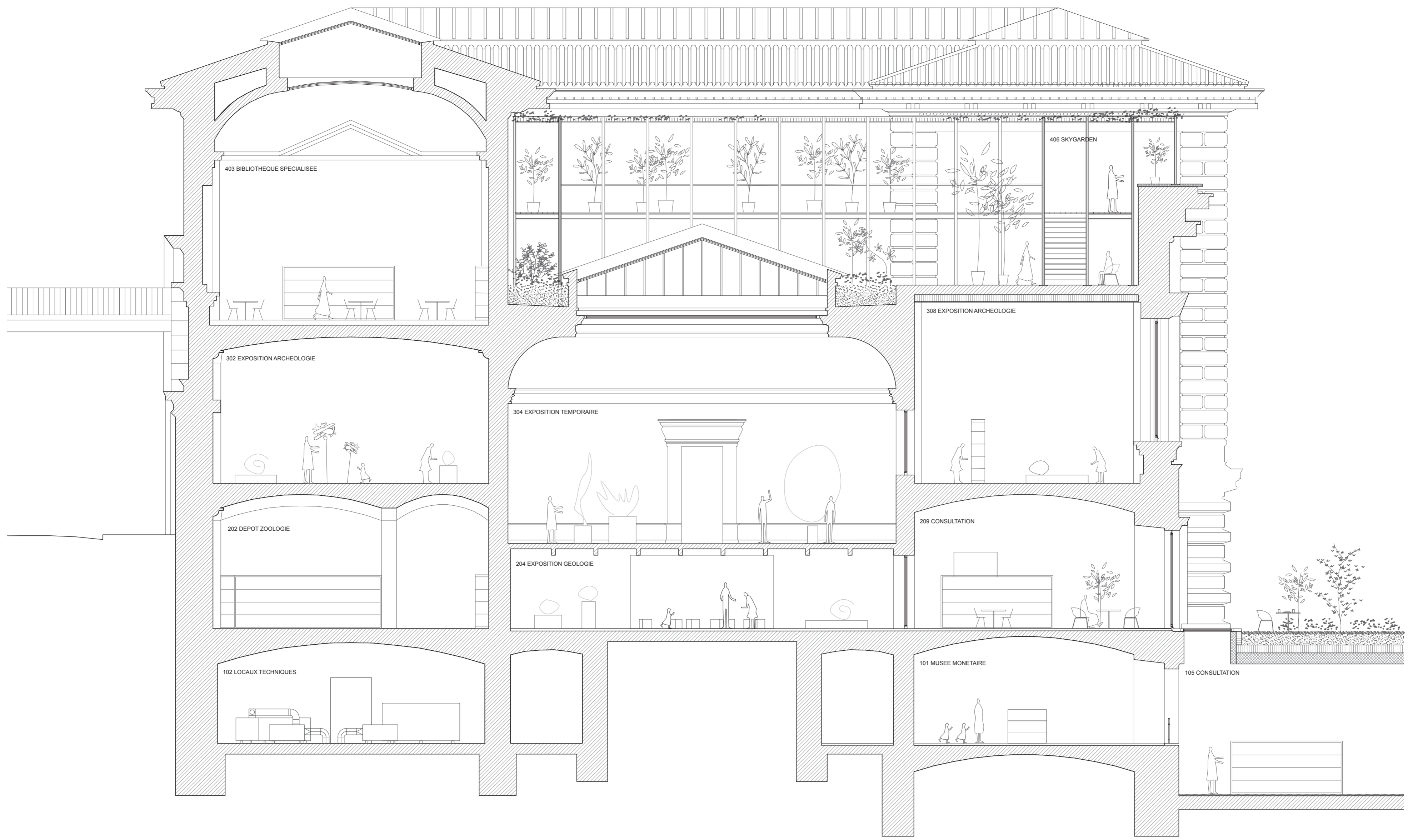
5 Coupe transversale nord 1:300
