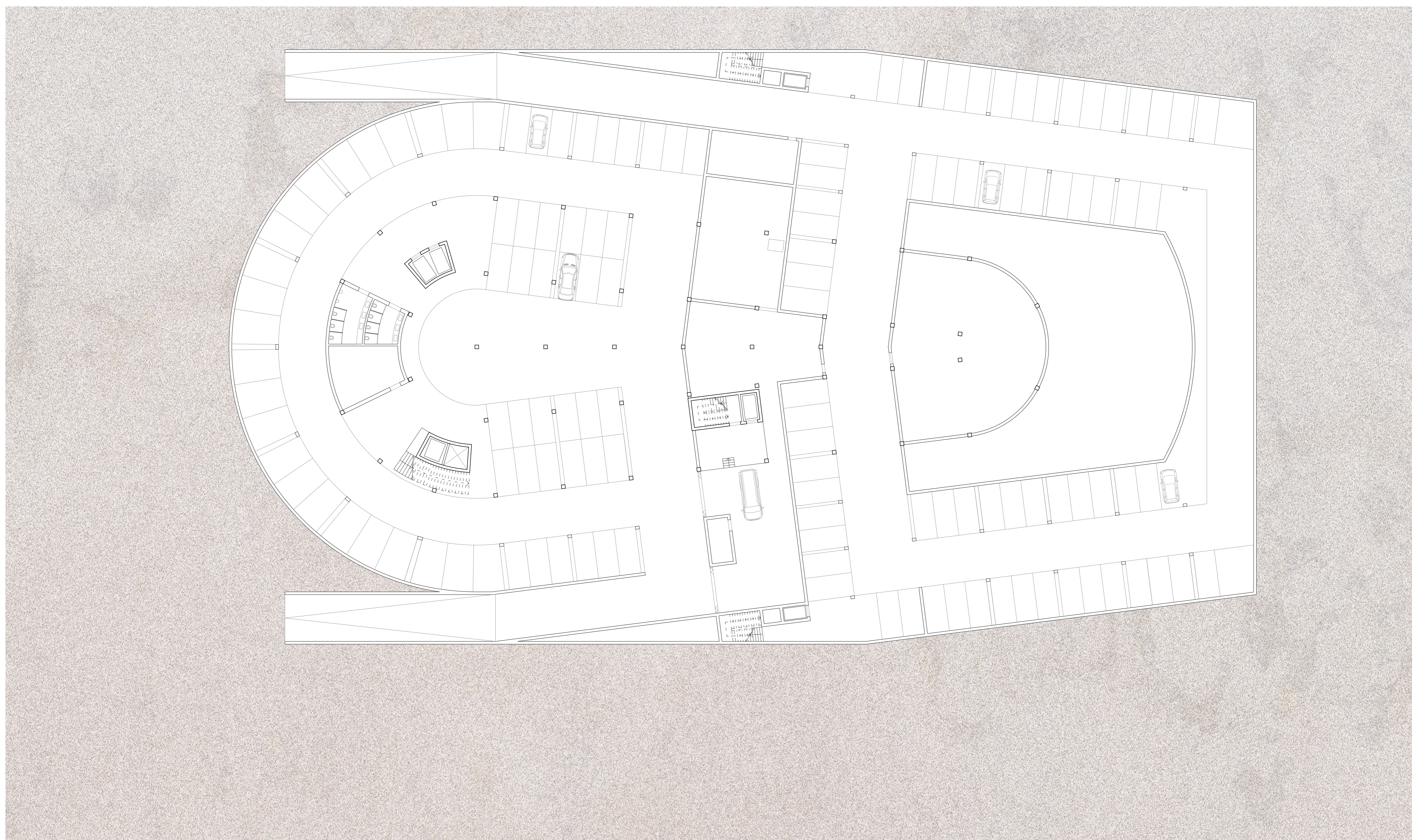
Plan du garage (niveau -1) 1/200
