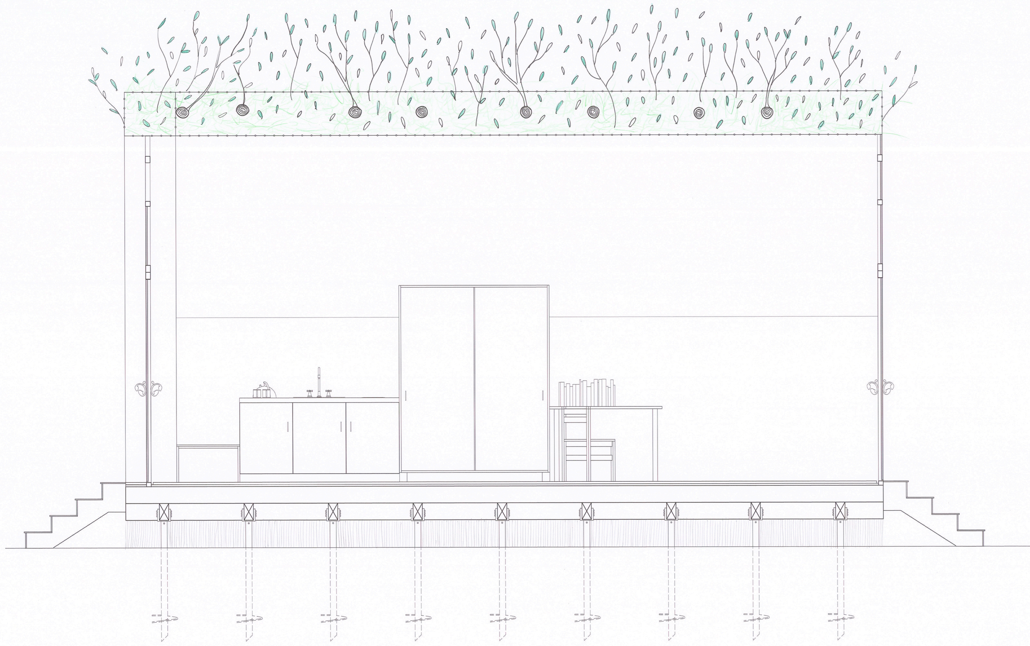
Coupe longitudinale 1:20
