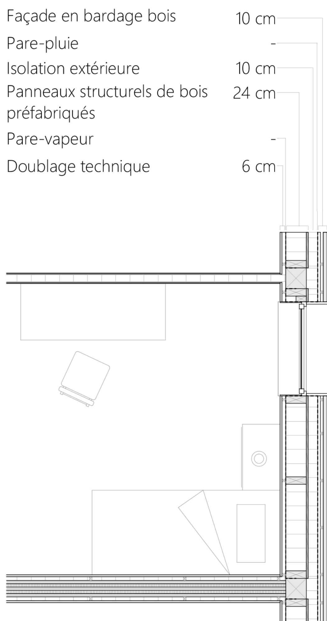
Détail façade nord / 1:25
