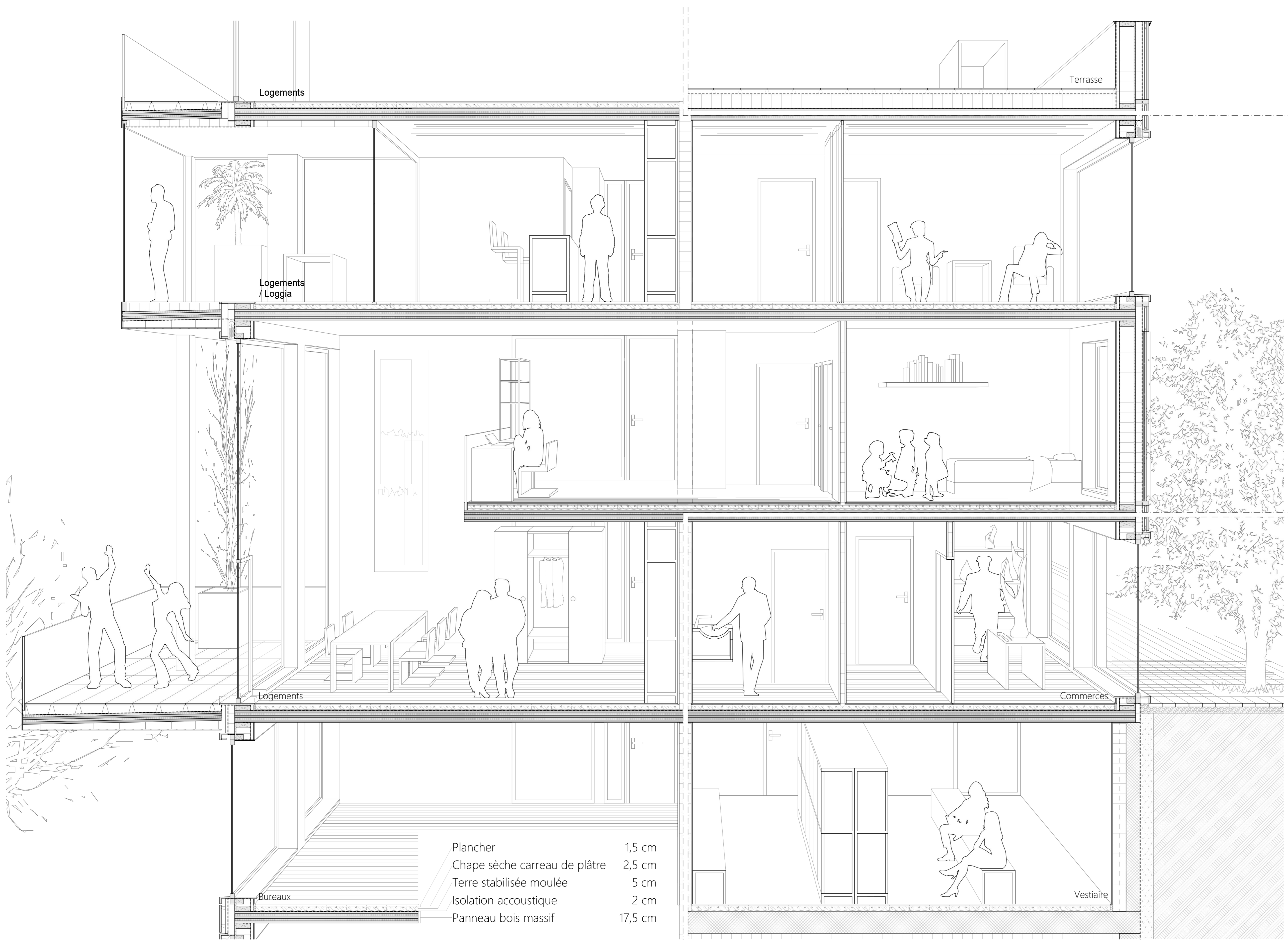
Coupe constructive en perspective / 1:25
