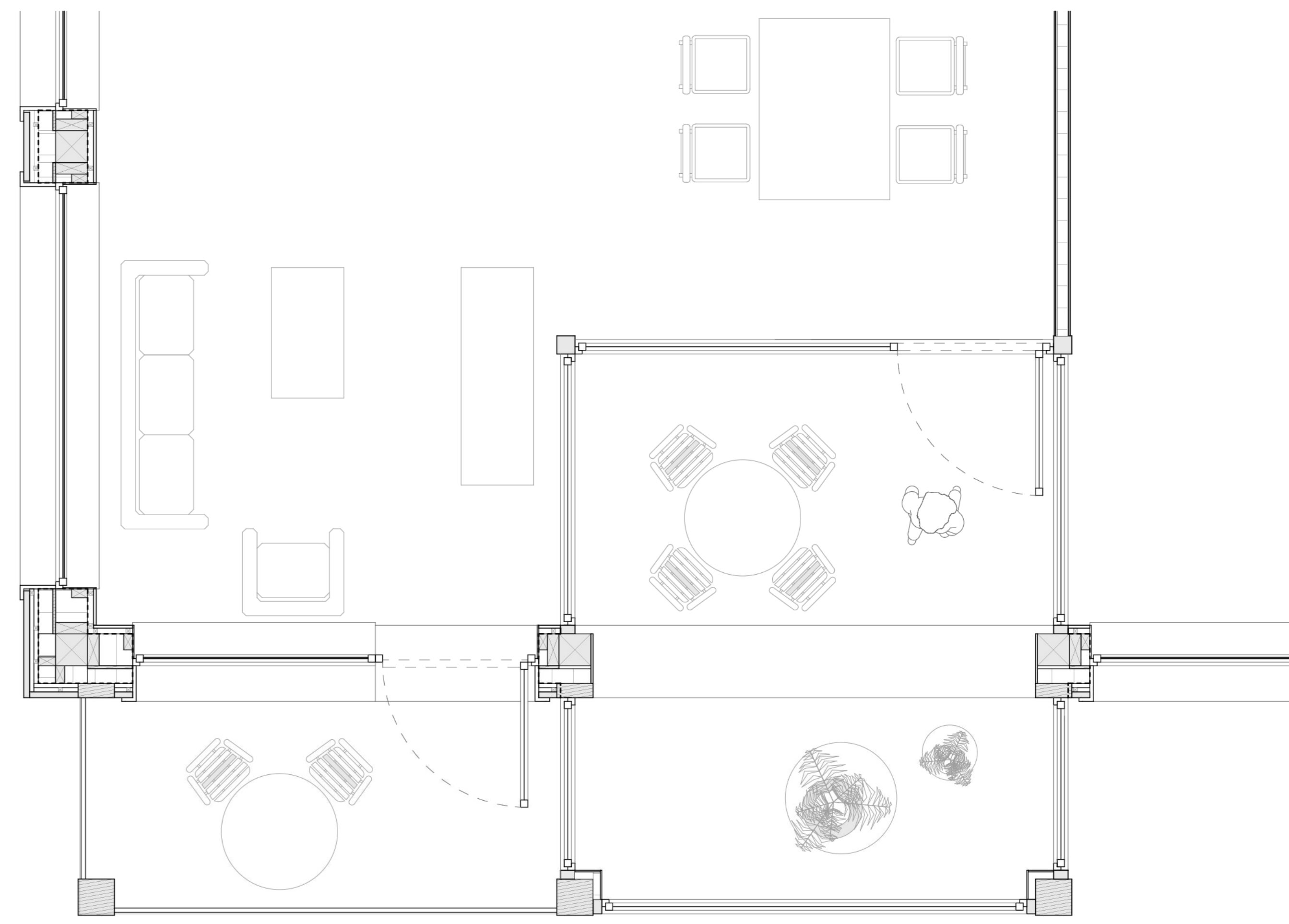
Détail façade sud / 1:25
