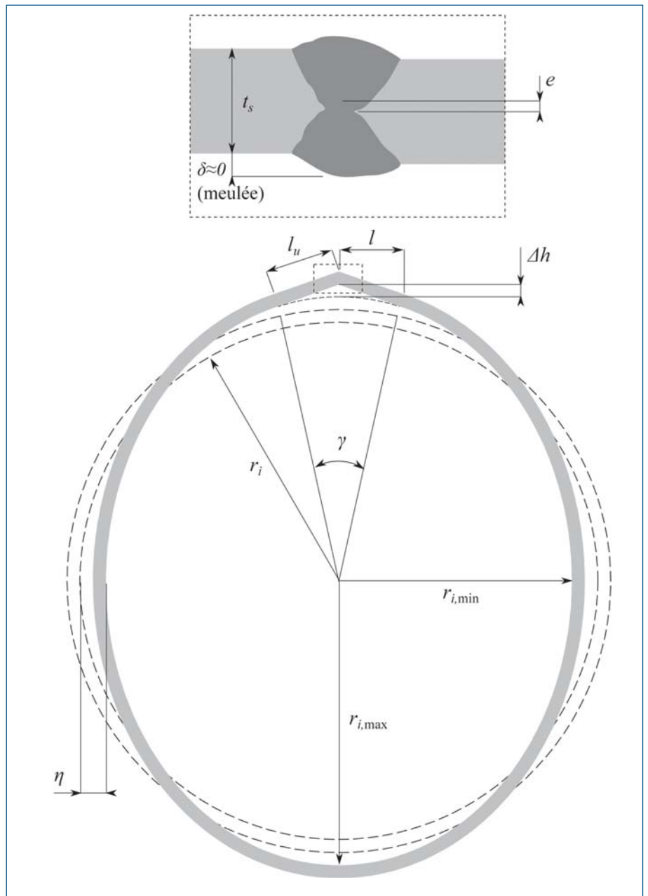
Figure 3. Schéma représentant les imperfections géométriques des viroles de blindage considérées dans cette étude.
