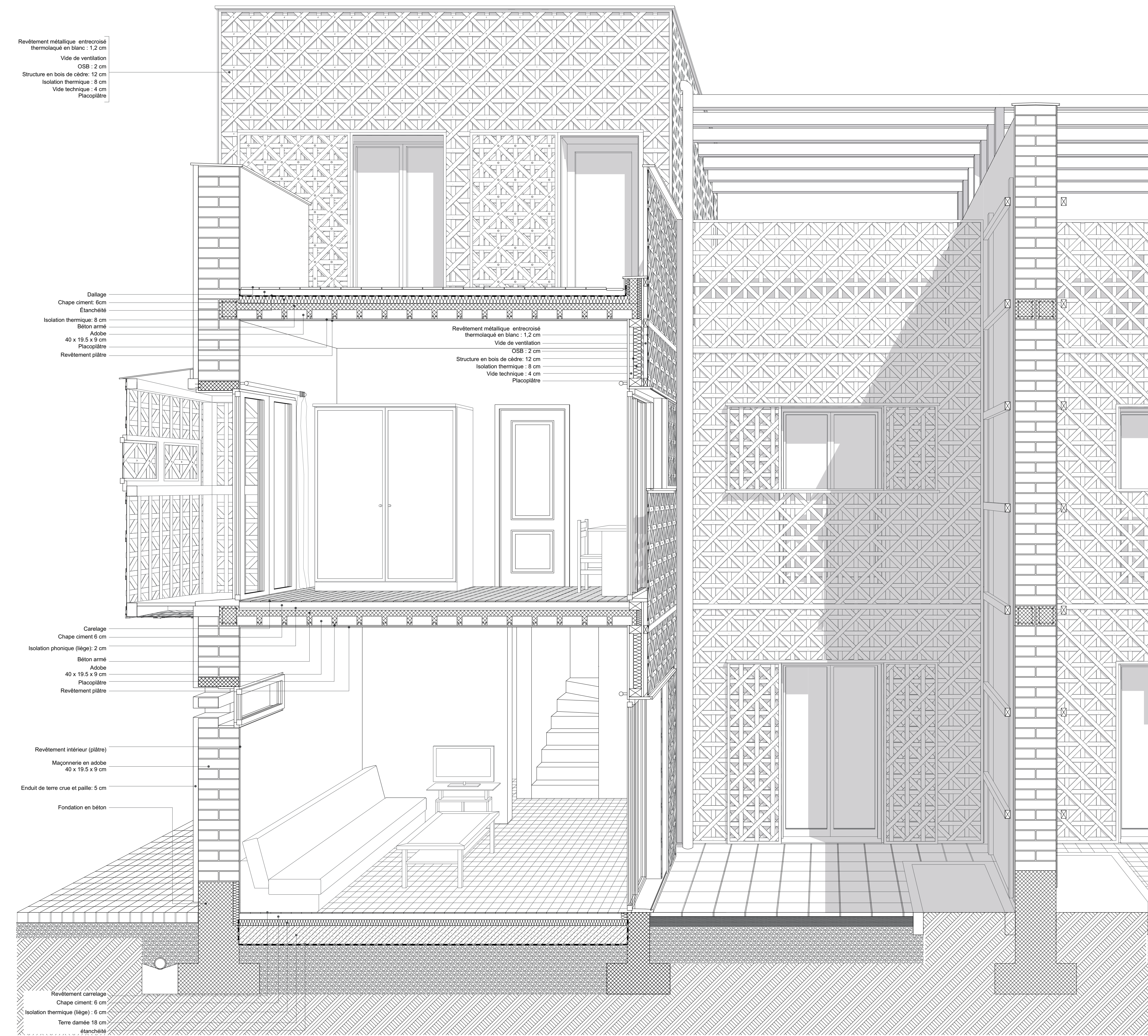
Détails 1:20
