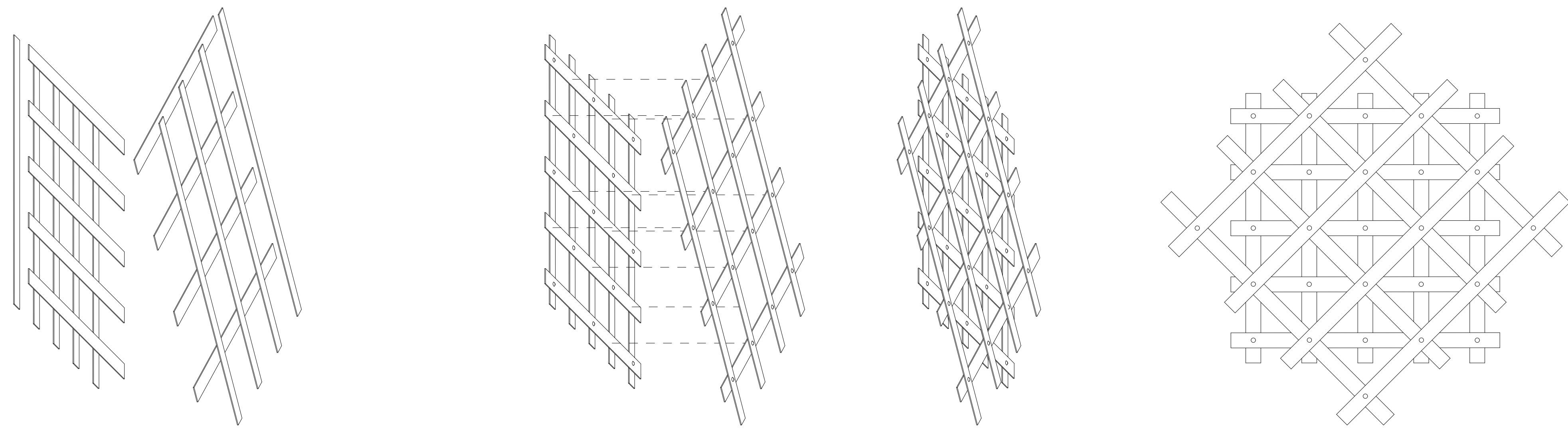
Détails du revêtement métallique entrecroisé 1:10 Assemblage de deux grilles orthogonales rivetées: méplats de 3mm d'épaisseur dans quatre directions
