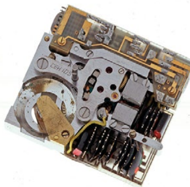
Fig. 6 : Calibre Beta 1, prototype de 1967. Photo : H. R. Bramaz.
