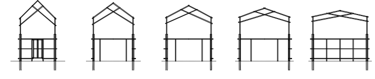
coupes: ensemble des fermes composantes 1:500
