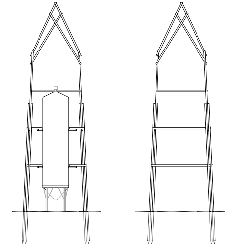
coupes: ensemble des fermes composantes 1:100
