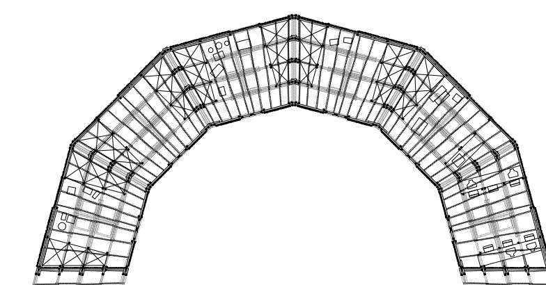
plan général 1:500
