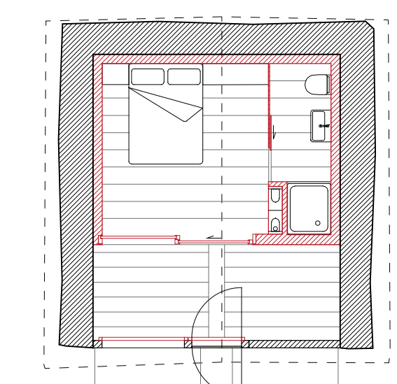
Plan : existant 25.3 m 2 , alcôve 13.9 m 2
