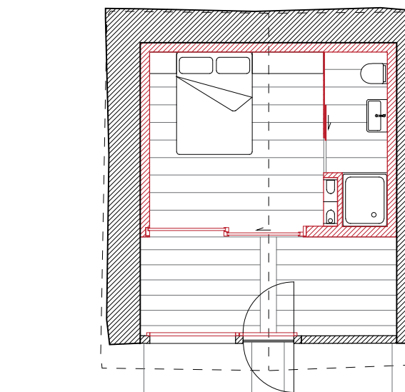
Plan : existant 25.8 m 2 , alcôve 14.3 m 2
