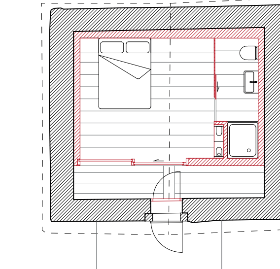
Plan : existant 23.3 m 2 , alcôve 15.5 m 2
