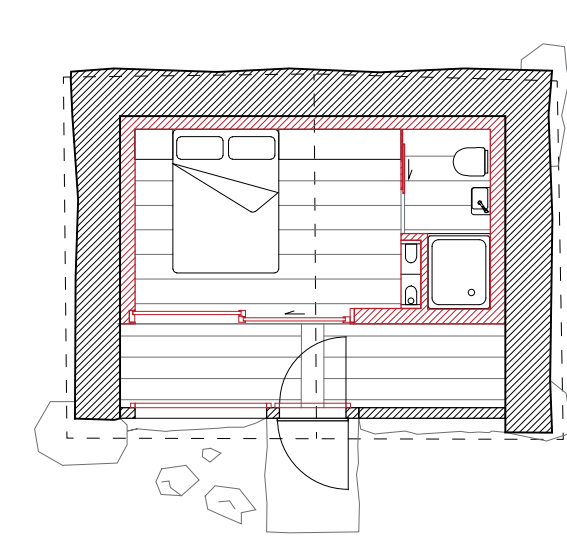
Plan : existant 19.7 m 2 , alcôve 11.2 m 2
