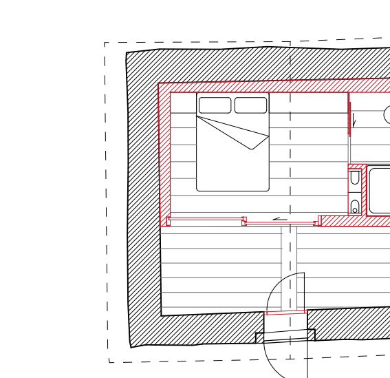
Plan : existant 22.2 m 2 , alcôve 11 m 2
