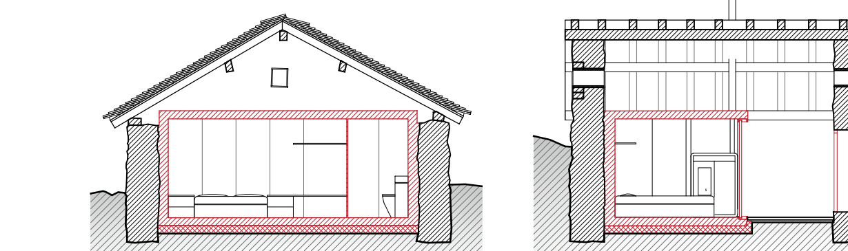
Coupe transversale Coupe longitudinale
