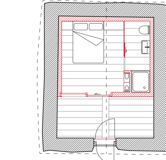
Plan : existant 24 m 2 , alcôve 12.9 m 2
