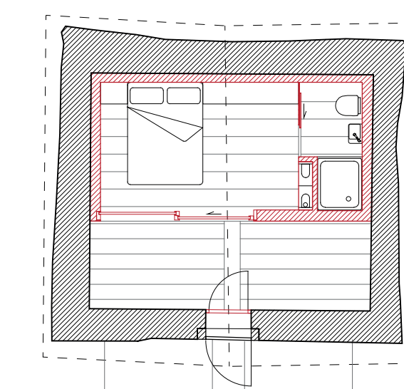
Plan : existant 22.9 m 2 , alcôve 11.6 m 2
