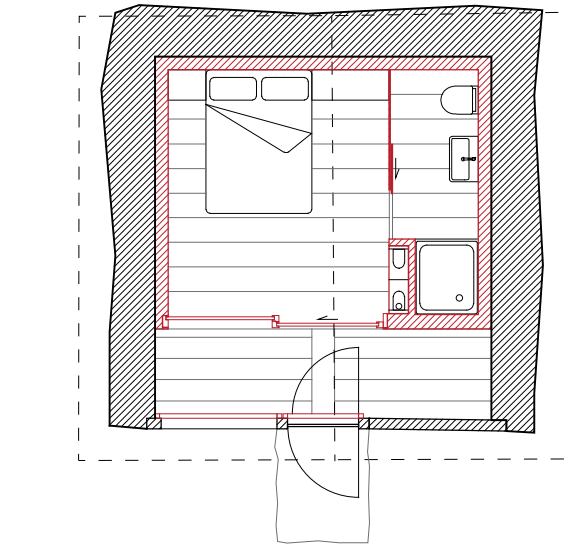
Plan : existant 21.3 m 2 , alcôve 13.3 m 2
