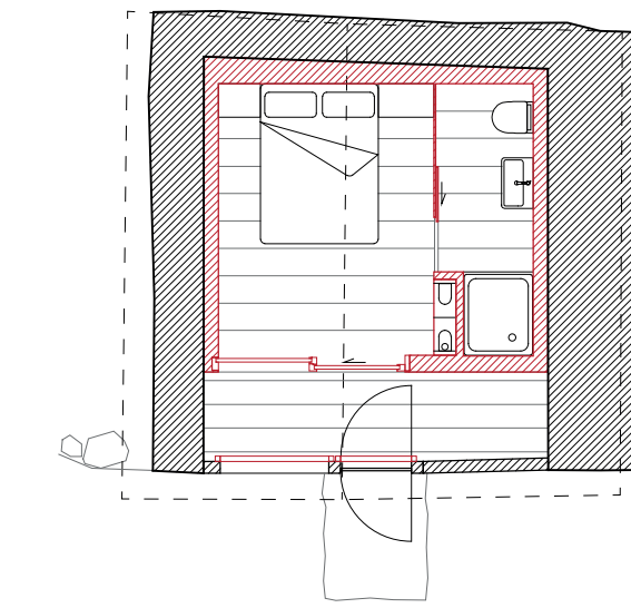
Plan : existant 31.9 m 2 , alcôve 12.1 m 2
