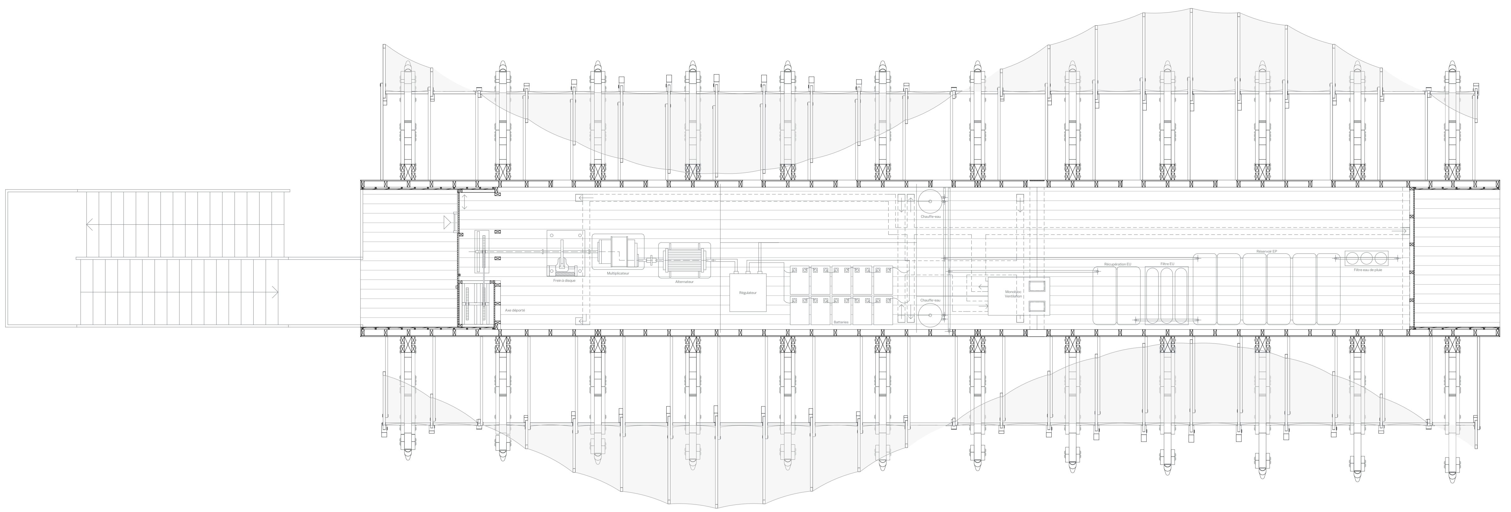
Plan. Machinerie.
