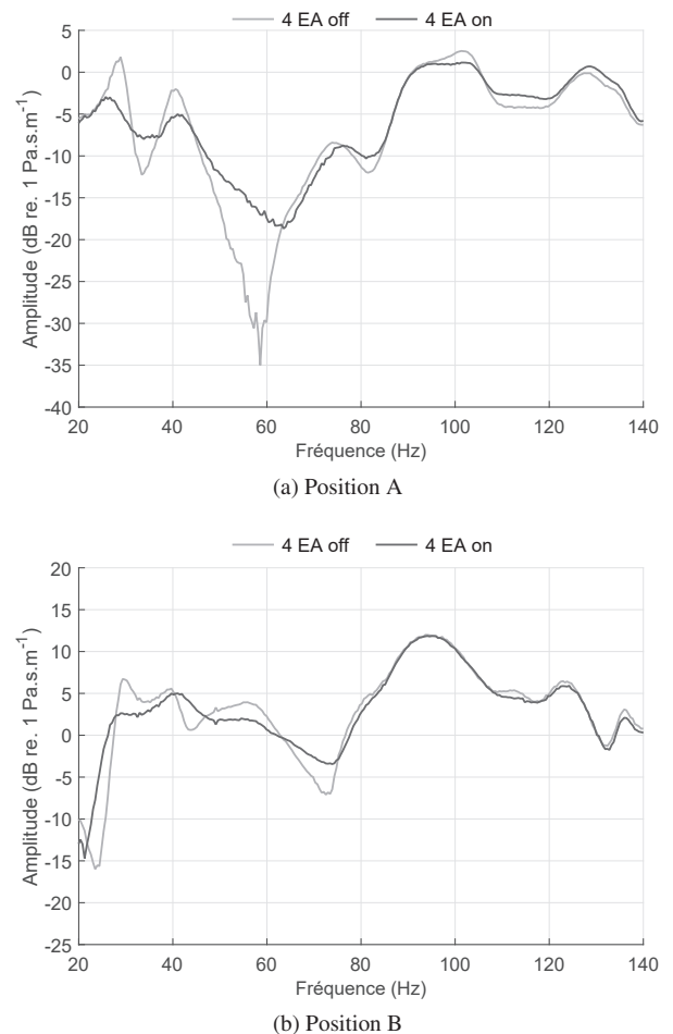
FIGURE 5 – Fonctions de transfert mesurées entre la vitesse de la membrane de la source sonore et le niveau de pression acoustique pour deux positions différentes dans la salle.
