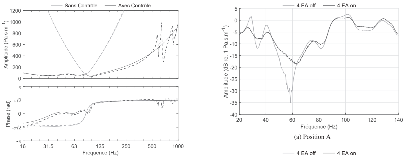
FIGURE 4 – Réponses en fréquence de l'impédance acoustique spécifique de l'absorbeur électroacoustique simulées (lignes continues) et mesurées (lignes pointillées) à l'extrémité d'un tube d'impédance avec et sans contrôle.
