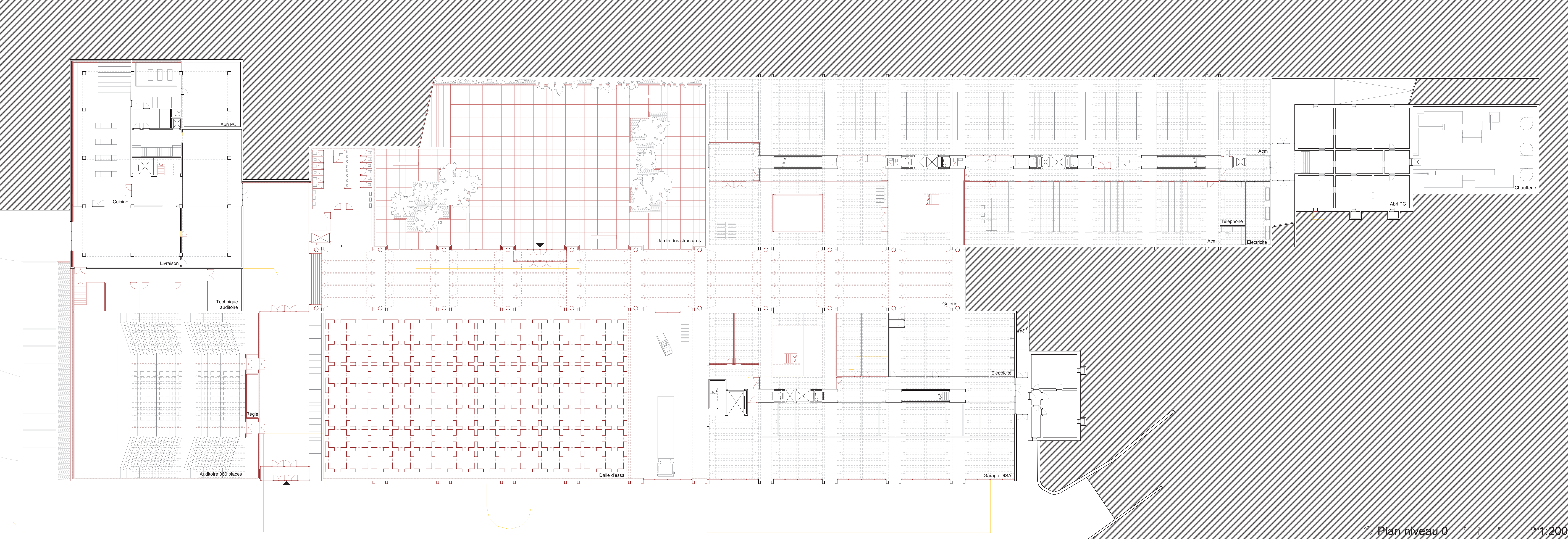
Plan niveau 1 0 1 2 5 10m 1:200
