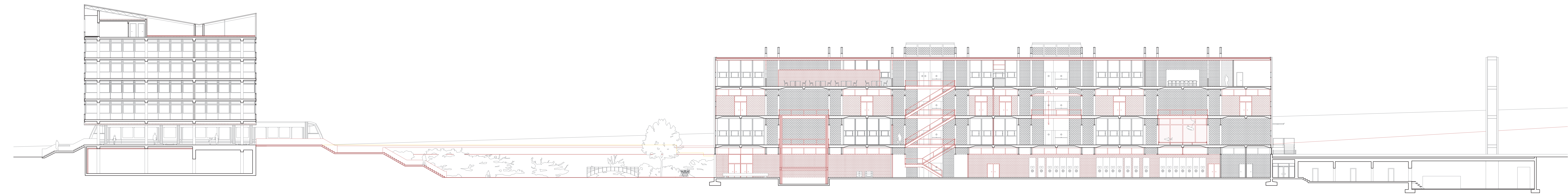
Coupe longitudinale bâtiments nord 0 1 2 5 10m 1:200
