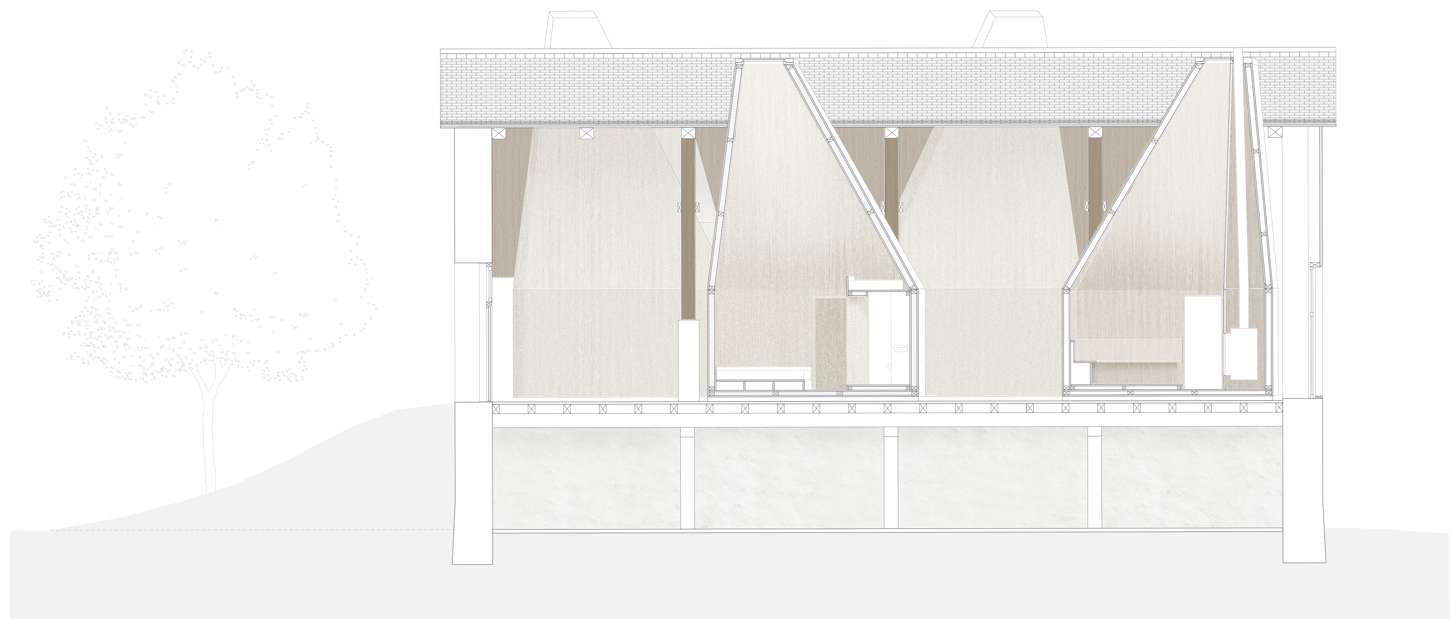
Coupe longitudinale | 1:50
