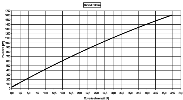
Fig. 3 Caratteristica d'uscita di una cella a combustibile di tipo PEM
