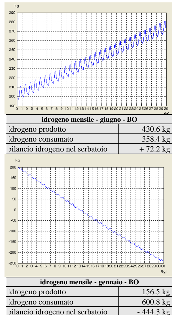
Fig. 10a,b Andamento mensile della quantità di idrogeno immagazzinata nel serbatoio nei mesi di giugno e gennaio
