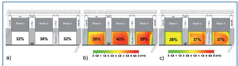
Figure 7. Vitesses d'écoulement et répartition du débit dans les trois pertuis du barrage, Q_{\text{Rhône}} = HQ_{\text{année 2000}} = 1270 \text{ m}^3/\text{s} , résultats de simulation a) avec Dunamic 2D, b) sur modèle physique et c) avec FLOW3D®.
