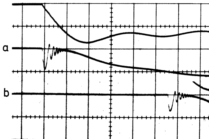
Fig. 3 a et b: Signal diamagnétique pour deux délais différents. 1,94 \mu\text{sec} / \text{div} .
