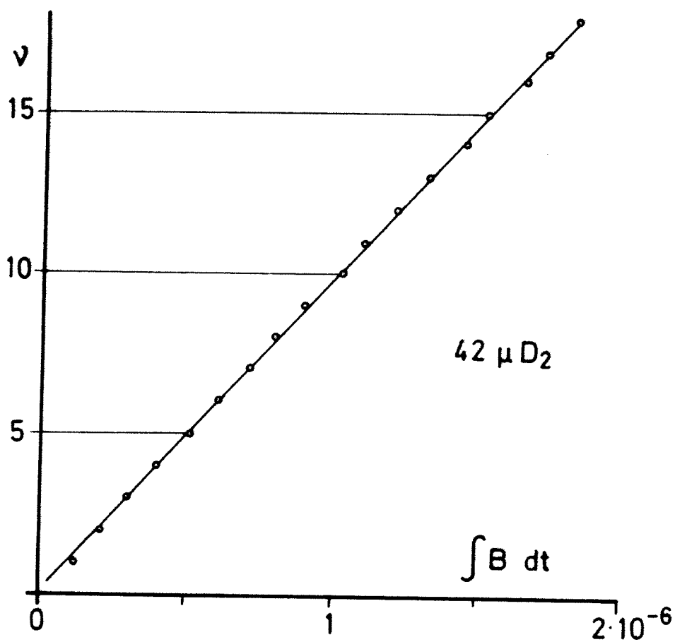
Fig. 5 Phase de l'oscillation radiale
