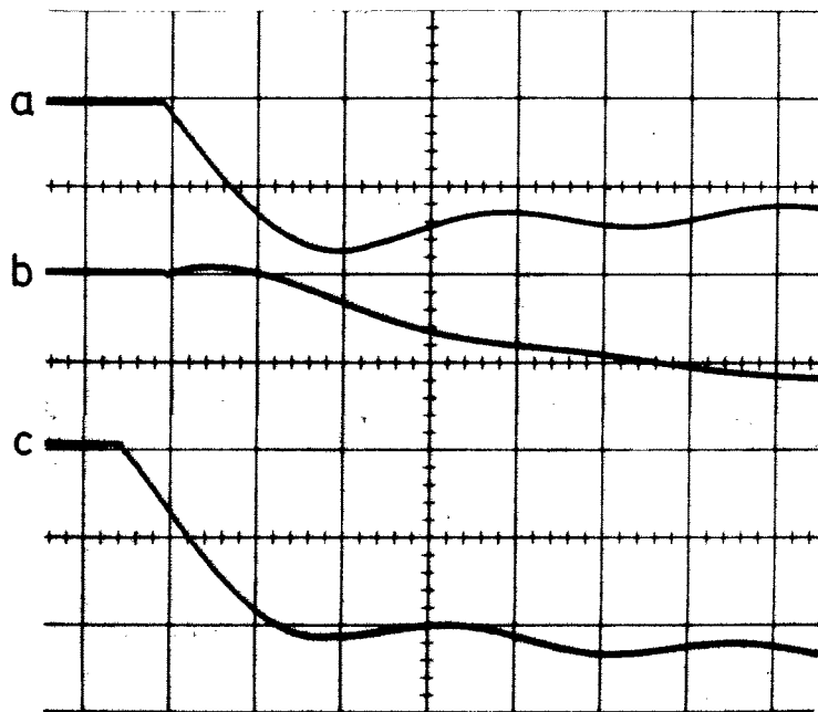
Fig. 2 a: champ magnétique. 1,94 \mu\text{sec} / \text{div} ; 9,6 \text{ kG} / \text{div} . b: signal zéro c: signal diamagnétique d'étalonnage
