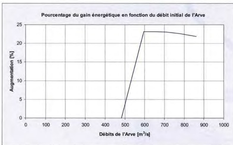
Fig. 7: Pourcentage du gain énergétique en fonction du débit initial de l'Arve.
