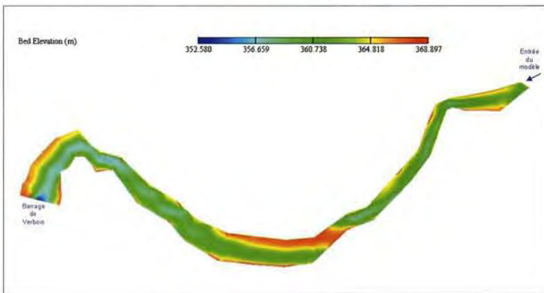
Fig. 9: Bathymétrie d'une partie de la retenue établie par CCHE2D.
