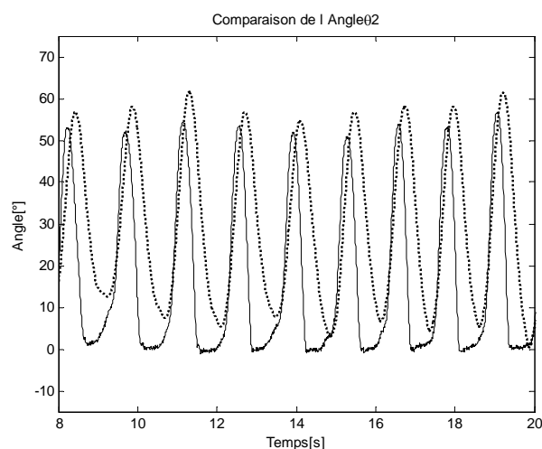
Figure3: Comparaison de la mesure de l'angle \theta_2 avec la méthode développée (trait discontinu) et un potentiomètre (trait continu) lors d'une marche de 3,5km/h
