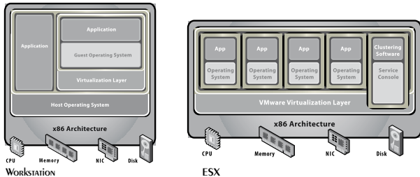
fig. 2 – ARCHITECTURE DE VIRTUALISATION
