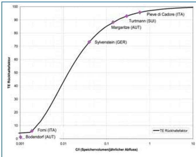
Bild 4. Rückhaltefaktor nach Brune (1953). Vergleich der Pilotprojekte im Rahmen des Projekts Interreg IIIB-Alpreserv.
