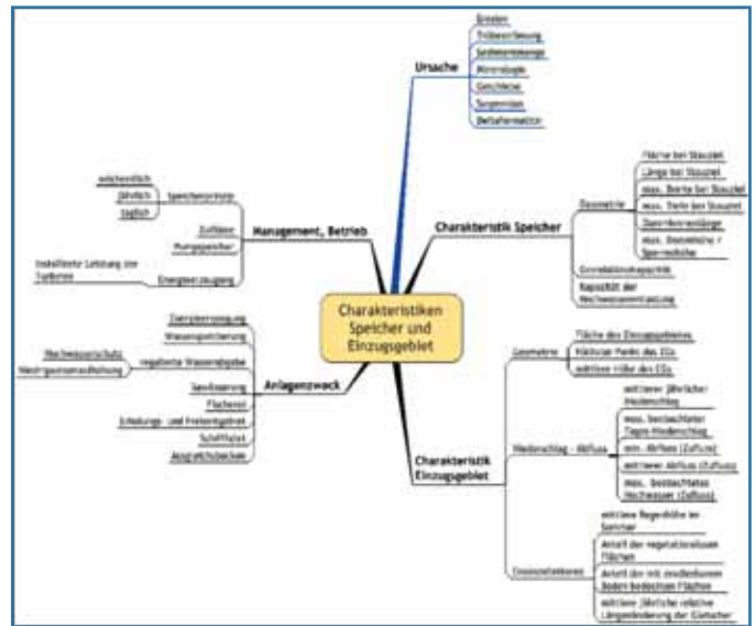
Bild 2. Parameter, die die Speicherverlandung beeinflussen.
