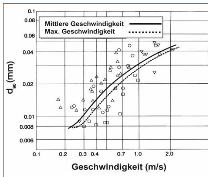
Bild 3. Maximal transportierbarer Korn-durchmesser in Abhängigkeit der Fließgeschwindigkeit des Trübestroms gemäss Fan (1986).
