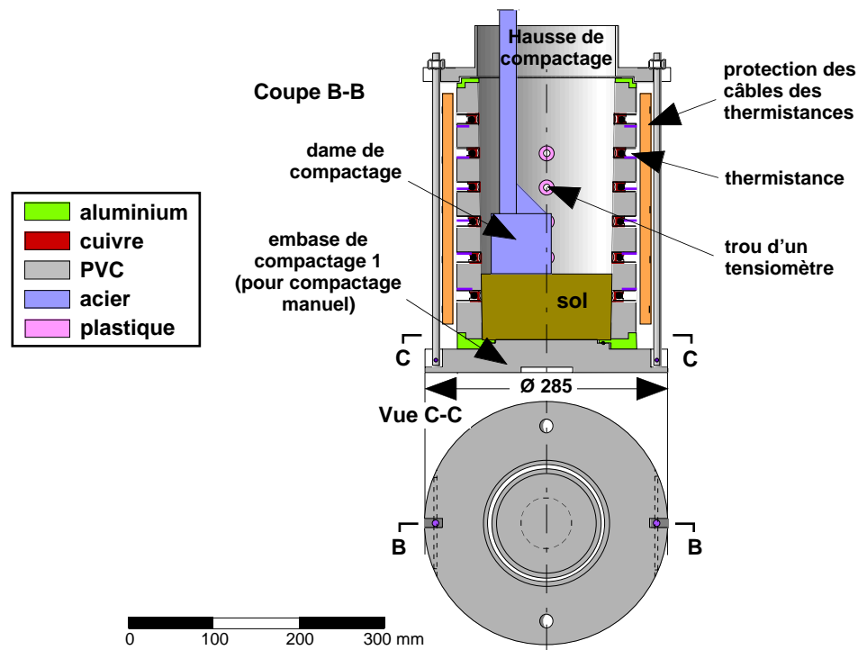
4-6 Le moule pendant le compactage manuel de l'éprouvette
