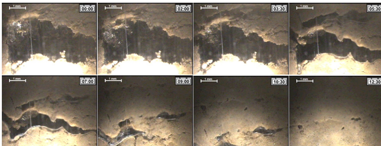
5-12 Essai no 3: Fonte d'une lentille, h=205 mm, 4 heures après début dégel, 0 h = 428 h (fig. 5-8). Séquence d'images tirée d'une animation.
